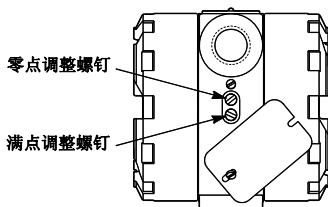
图 4. 零点和满点的调整螺钉
