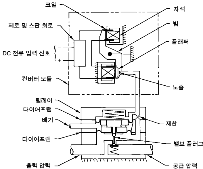
그림 8. Fisher 646 트랜스듀서 설계도
