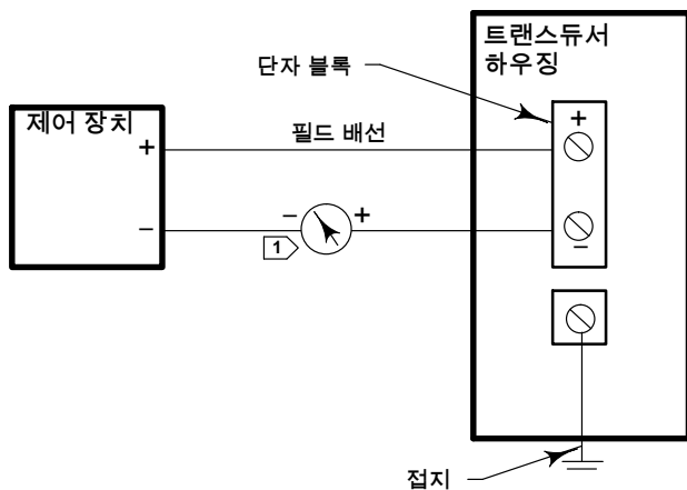
그림 5. 일반 필드 배선 도해
