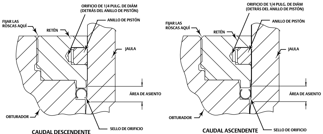
Figura 3. Válvula Fisher ED/EWD equipada con el sello de orificio
