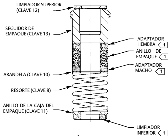
Figura 2. Empaque típico
