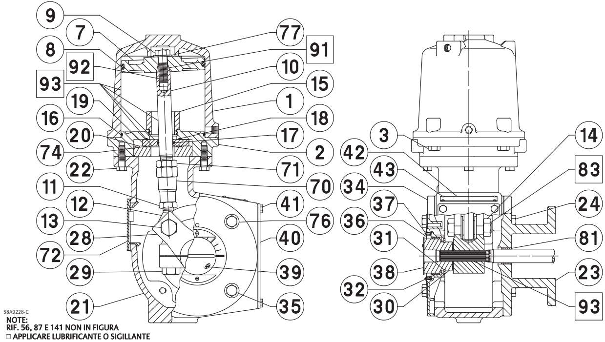
Figura 9. Montaggio tipico per attuatori Fisher 1061 dimensioni 80 a 100
