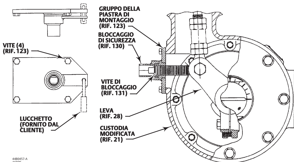
Figura 6. Meccanismo di bloccaggio (dimensioni 80 e 100)
