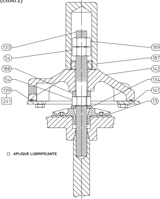
Figura 20. Batente de Deslocamento Ajustável para Baixo Montado na Caixa para Actuadores de Tamanhos 30/30i e 40/40i (Estilo 2)
