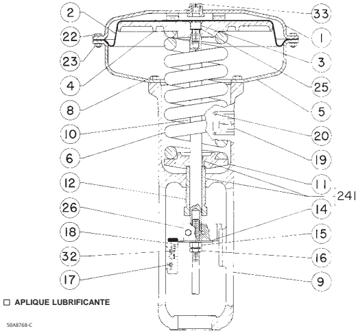
Figura 8. Actuador 657 de Tamanho 70 da Fisher
