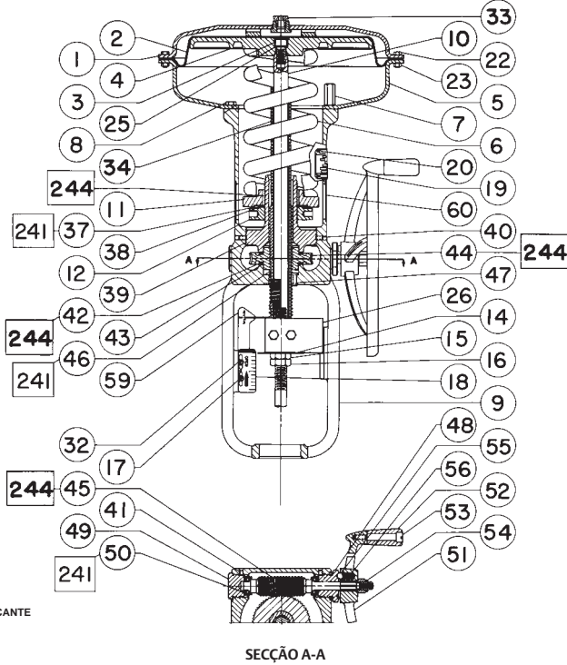
Figura 17. Actuadores 657 de Tamanhos 70 e 87 da Fisher com Volante Montado no Lado
