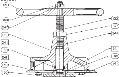
Figura 11. Conjunto de Volante Montado na Parte Superior para Actuadores de Tamanhos 30/30i a 60/60i
