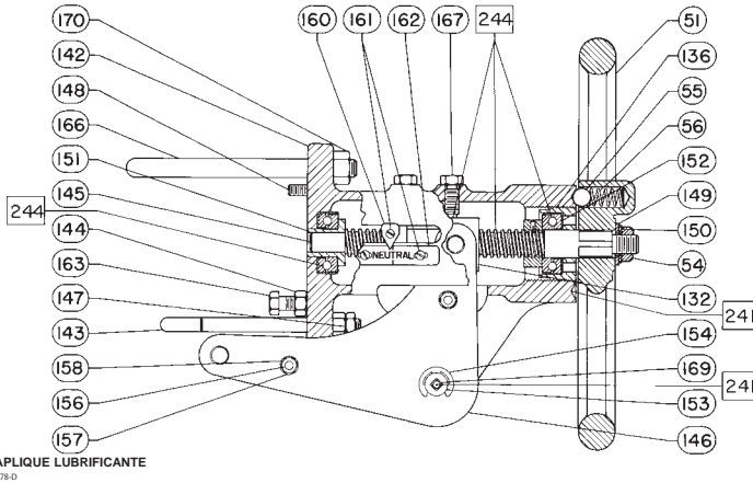
Figura 13. Conjunto de Volante Montado no Lado para Actuadores de Tamanhos 34 e 40
