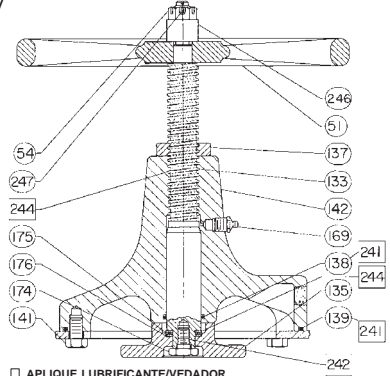
Figura 12. Conjunto de Volante Montado na Parte Superior para Actuadores de Tamanhos 70/70i a 87
