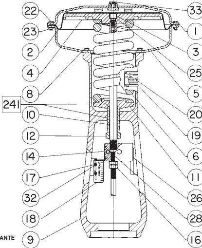
Figura 10. Actuador 657 de Tamanho 87 da Fisher
