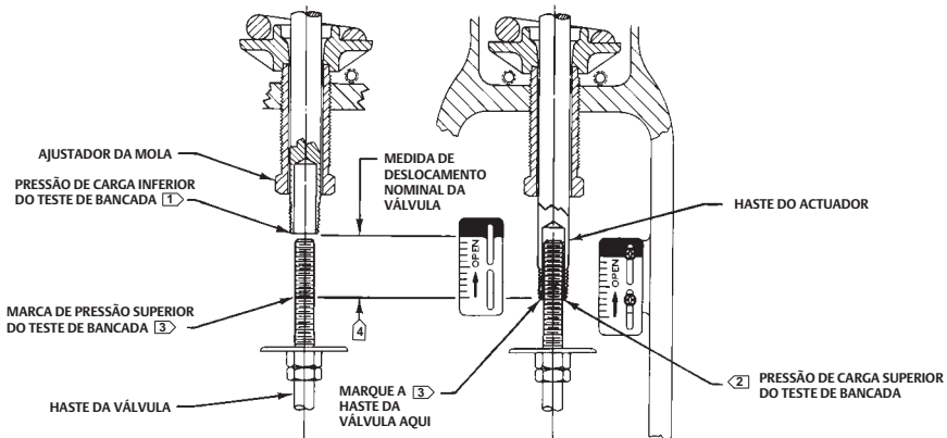
Figura 4. Ajuste do Teste de Bancada
