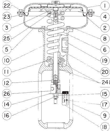
Figura 6. Actuador 657 de Tamanhos 30 a 60 da Fisher
