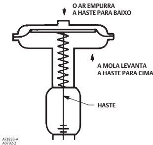
Figura 2. Esquemática dos Actuadores 657 e 657-4 da Fisher
