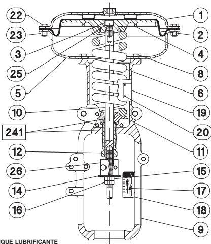
Figura 7. Actuador 657 de Tamanhos 30i a 60i da Fisher
