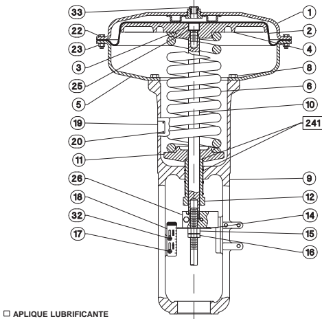
Figura 9. Actuador 657 de Tamanho 70i da Fisher
