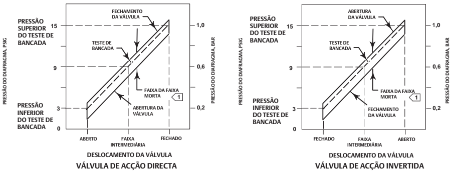
Figura 5. Resposta Típica da Válvula à Faixa Morta
