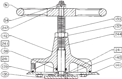
Figure 11. Montage du volant supérieur des actionneurs de tailles 30/30i à 60/60i
