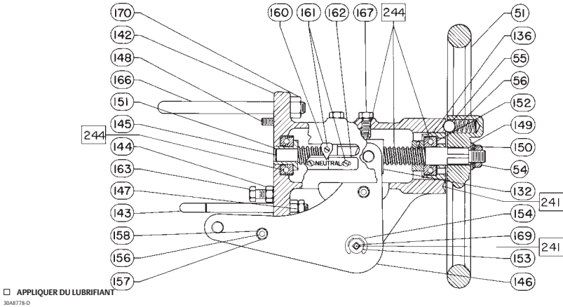
Figure 13. Volant latéral des actionneurs de tailles 34 et 40
