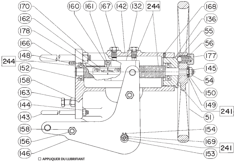
Figure 15. Volant latéral des actionneurs de tailles 45, 46, 50 et 60
