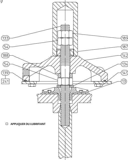
Figure 20. Butée de course descendante réglable montée sur boîtier pour actionneurs de tailles 30/30i et 40/40i (Style 2)
