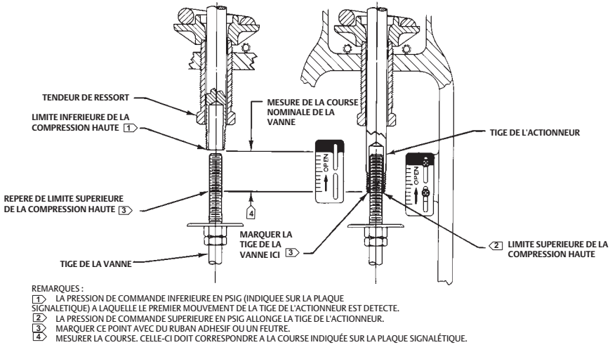
Figure 4. Réglages de la compression
