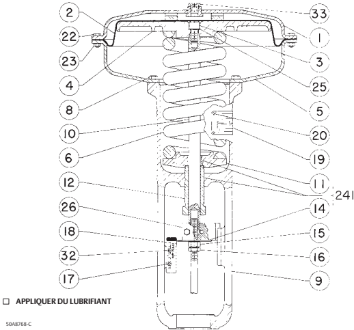
Figure 8. Actionneur Fisher 657, taille 70
