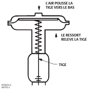
Figure 2. Schéma des actionneurs Fisher 657 et 657-4
