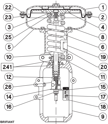
Figure 7. Actionneurs Fisher 657, de tailles 30i à 60i
