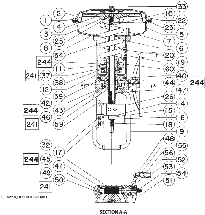
Figure 17. Actionneurs Fisher 657 de tailles 70 et 87 volant latéral
