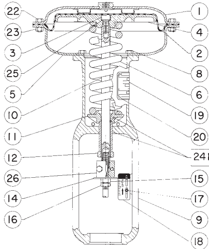
Figure 6. Actionneur Fisher 657, tailles 30 à 60
