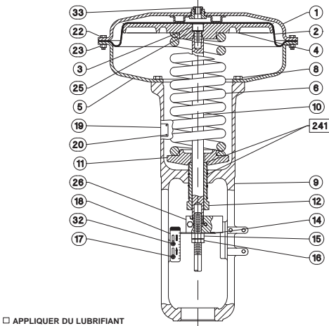
Figure 9. Actionneur Fisher 657, de taille 70i
