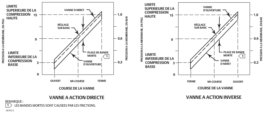
Figure 5. Réponse typique d'une vanne aux bandes mortes
