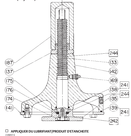
Figure 19. Butée de course ascendante réglable montée sur boîtier pour actionneurs de tailles 70/70i et 87 (Style 1)
