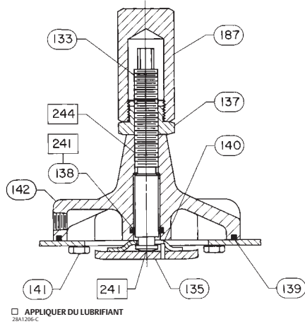
Figure 18. Butée de course ascendante réglable montée sur boîtier pour actionneurs de tailles 30/30i à 60/60i (Style 1)
