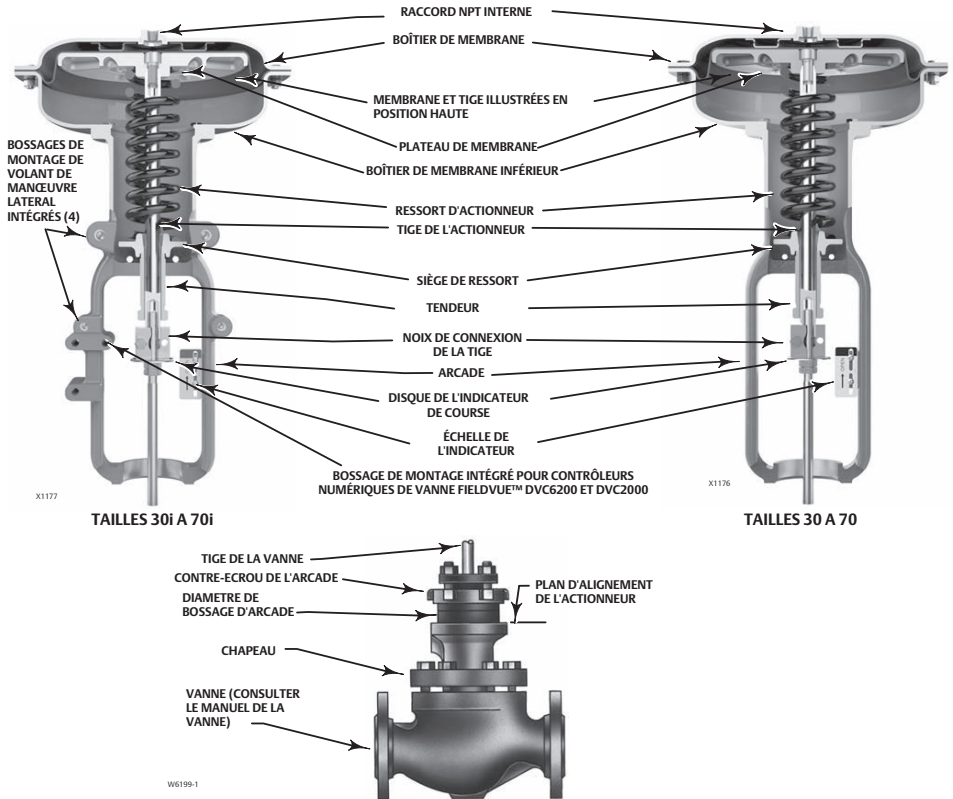
Figure 3. Composants de montage des actionneurs de tailles 30/30i à 70/70i
