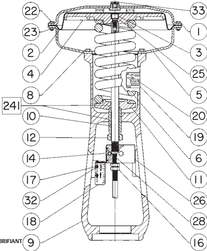
Figure 10. Actionneur Fisher 657, taille 87
