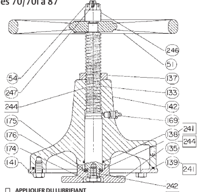
Figure 12. Montage de la commande manuelle montée en position supérieure des actionneurs de tailles 70/70i à 87
