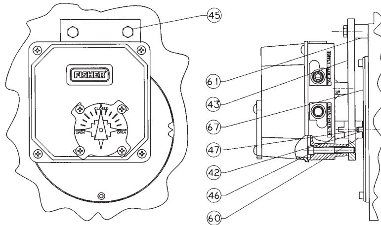
POSICIONADOR 3710 MONTADO EM UM ATUADOR 1031 DE TAMANHOS 20 A 80
