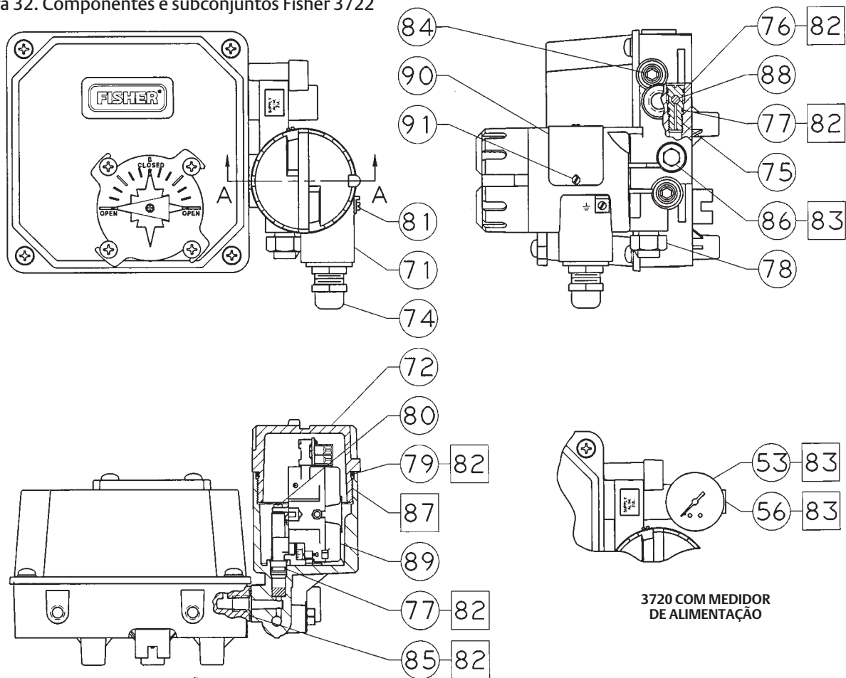
Figura 32. Componentes e subconjuntos Fisher 3722
