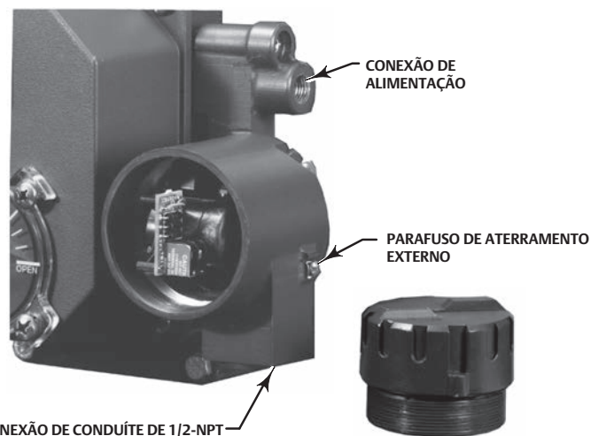
Figura 3. Conversor eletropneumático 3722 da Fisher
