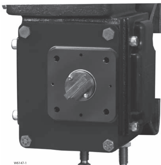
BARRA DO TIRANTE, PLACA DE MONTAGEM REMOVIDA
