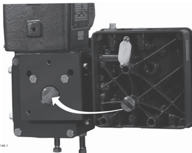
VISTA TRASEIRA, PLACA DA BASE DO POSICIONADOR E ÁREA DE MONTAGEM
