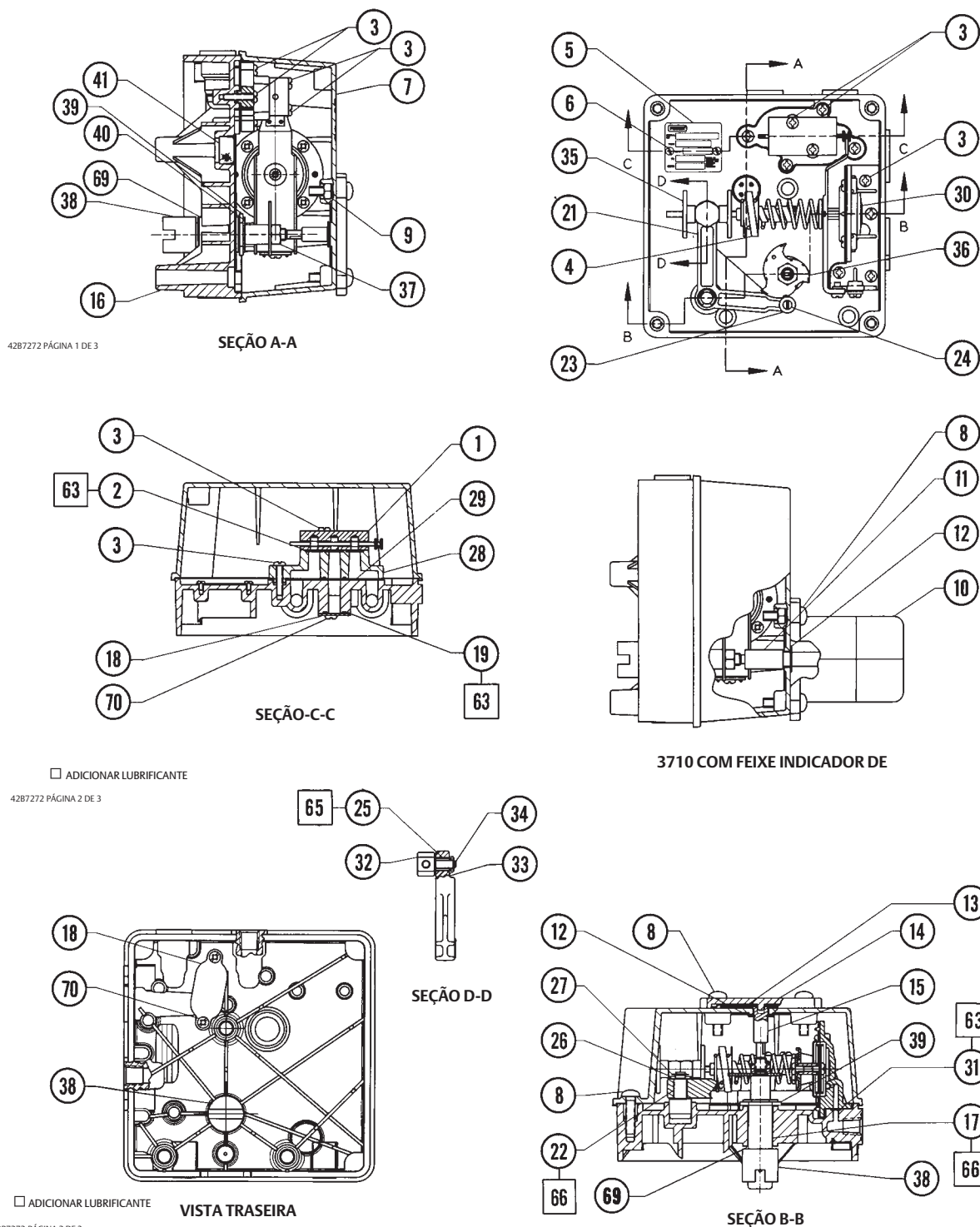
Figura 31. Componentes e subconjuntos Fisher 3710
