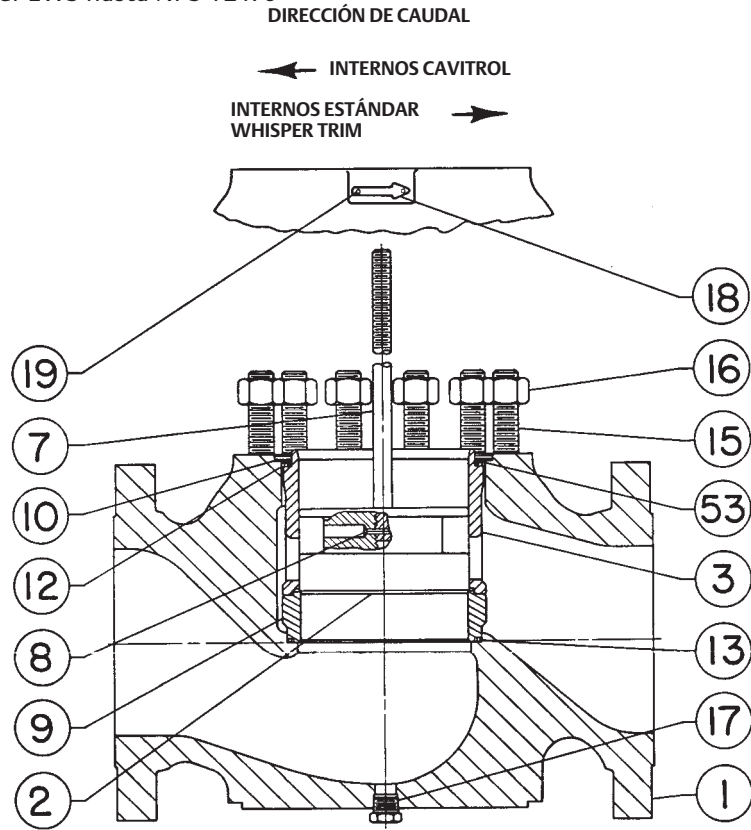
CONJUNTO COMPLETO DE VÁLVULA CON ASIENTO METÁLICO Y TAPÓN DE DRENAJE OPCIONAL
