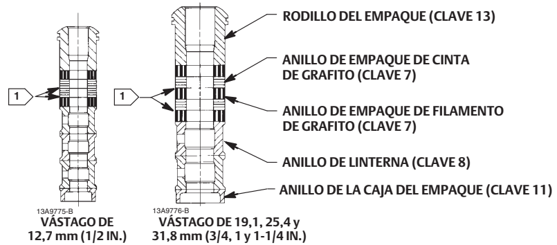
Figura 6. Detalle de cinta de grafito/empaque de filamento
