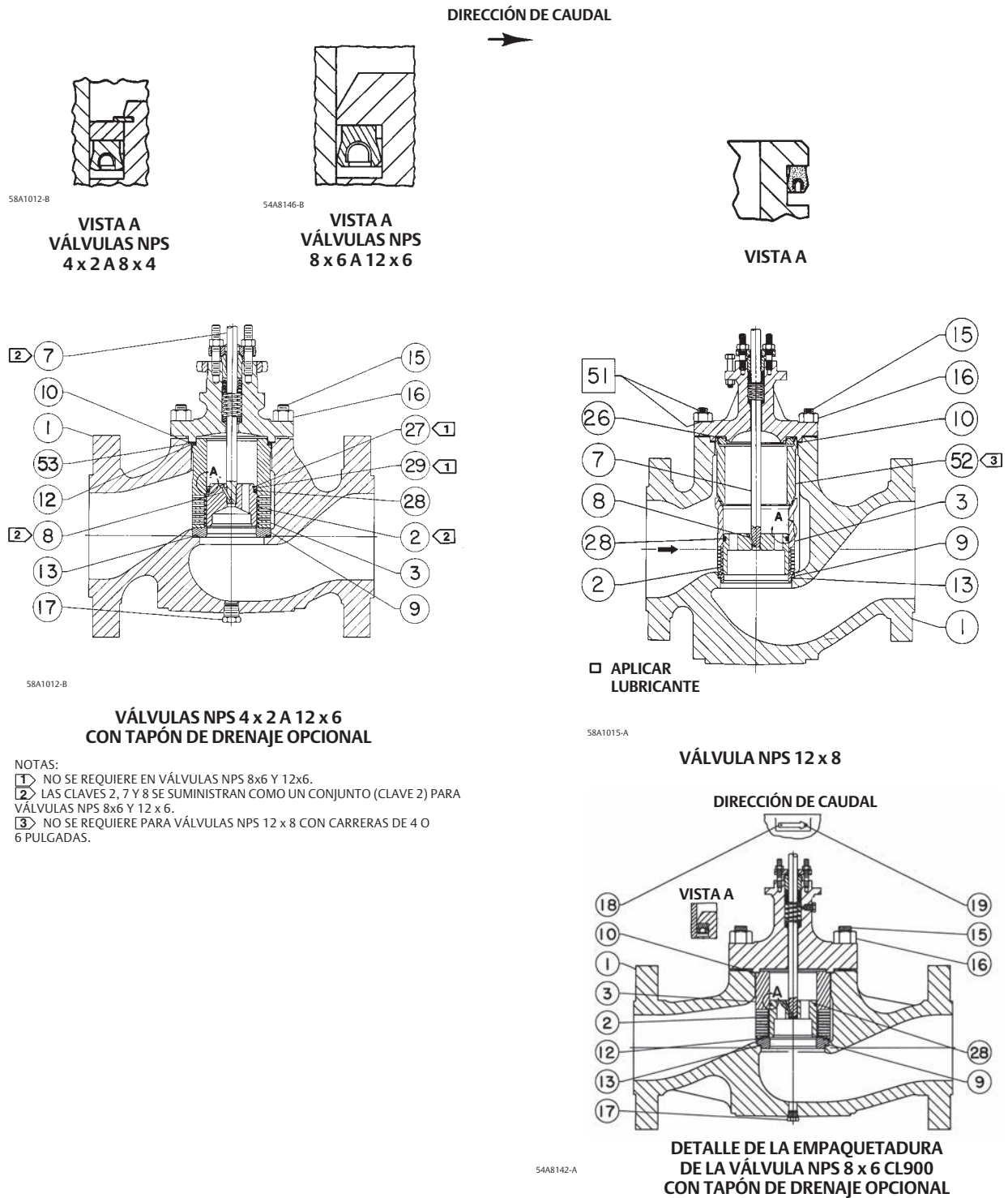
Figura 26. Válvula Fisher NPS 4x2 a 12x8 con jaula Cavitol III de una etapa
