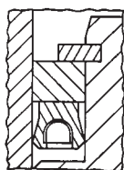
VISTA A
