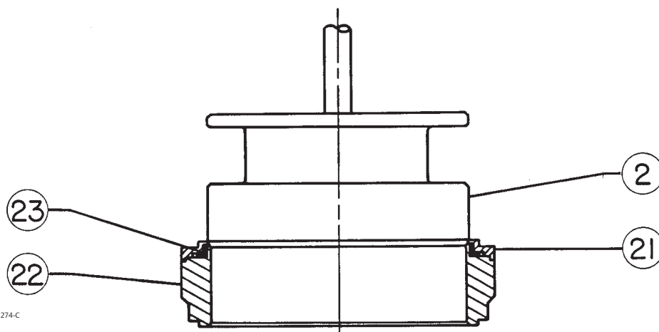
DETALLE DEL ASIENTO DE ELASTÓMERO
