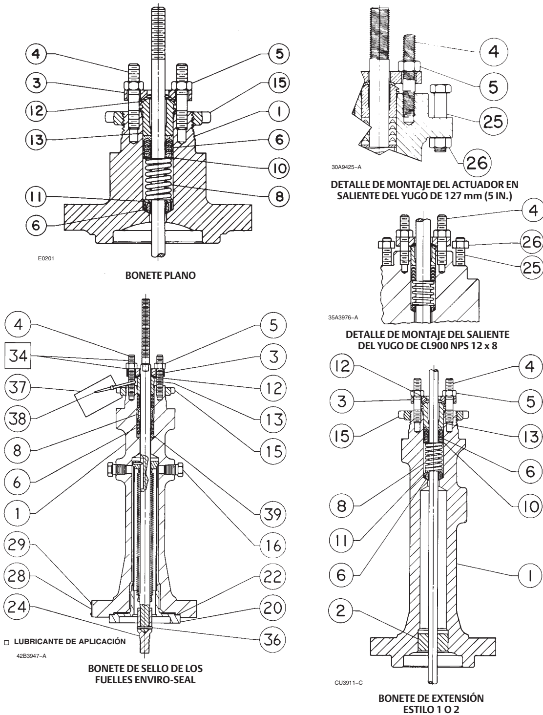
Figura 21. Bonete típico Fisher con conjunto de empaque de anillo V de PTFE individual
