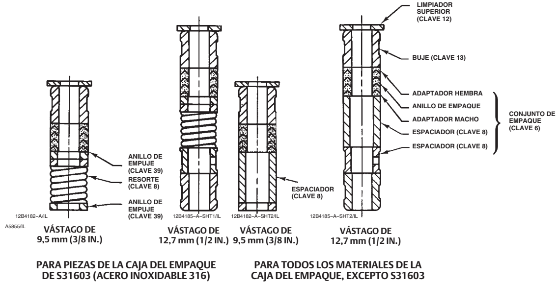
Figura 15. Arreglo de empaque de PTFE para bonetes de sello de fuelles Fisher ENVIRO-SEAL
