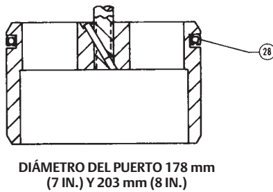
A2069-2 DETALLES DEL TAPÓN DE VÁLVULA CON ANILLO DE SELLO Y CARGA EN EL RESORTE
