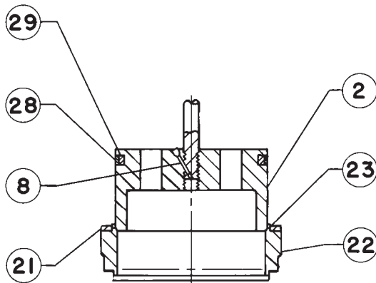
43A8590-B DETALLE DEL ASIENTO DE PTFE Y DEL TAPÓN DE VÁLVULA CON ANILLO DE SELLO DE 2 PIEZAS
