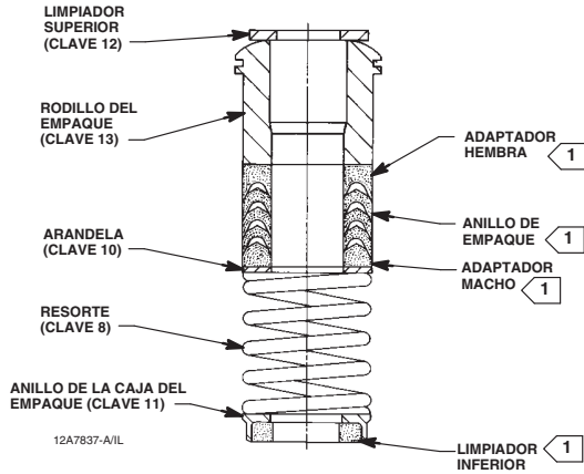
Figura 4. Arreglos de empaque de anillo V de PTFE
