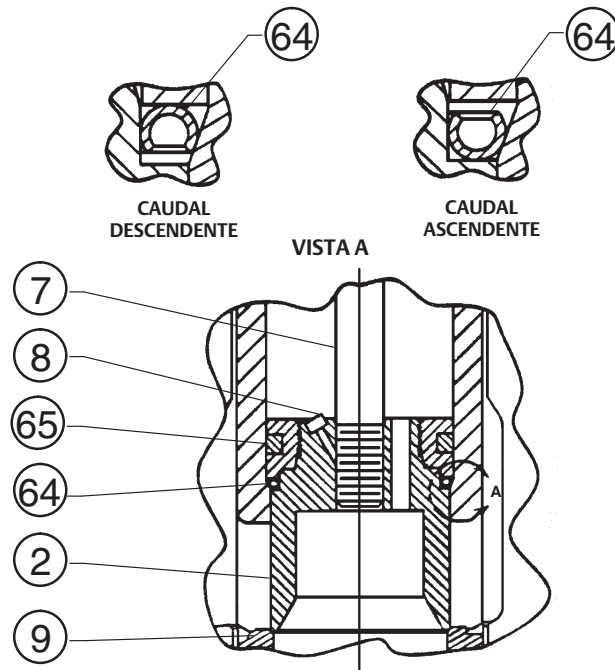
Figura 9. Fisher EWD con internos C-seal
