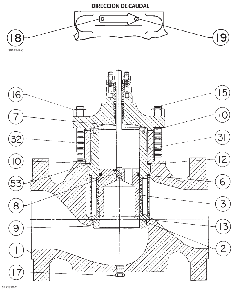
CONJUNTO COMPLETO DE VÁLVULA CON JAULA WHISPER TRIM III, ANILLO DE PISTÓN DE GRAFITO INDIVIDUAL Y TAPÓN DE DRENAJE OPCIONAL
