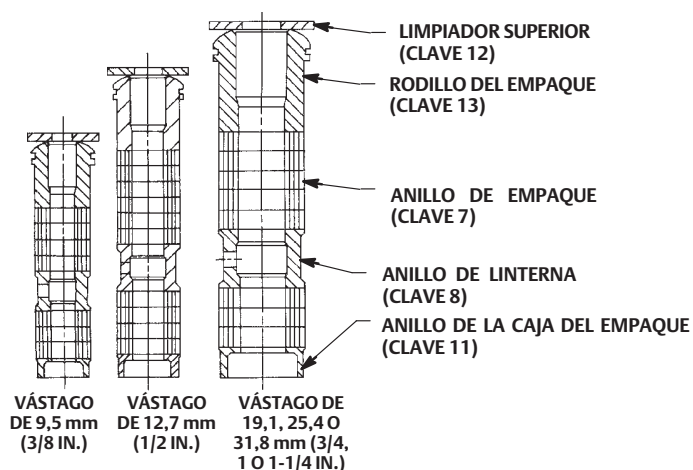
Figura 5. Detalle de los arreglos de empaque de PTFE/composición
