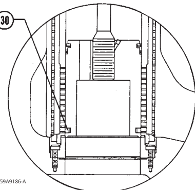
DETAIL DU WHISPER TRIM DE NIVEAU D
