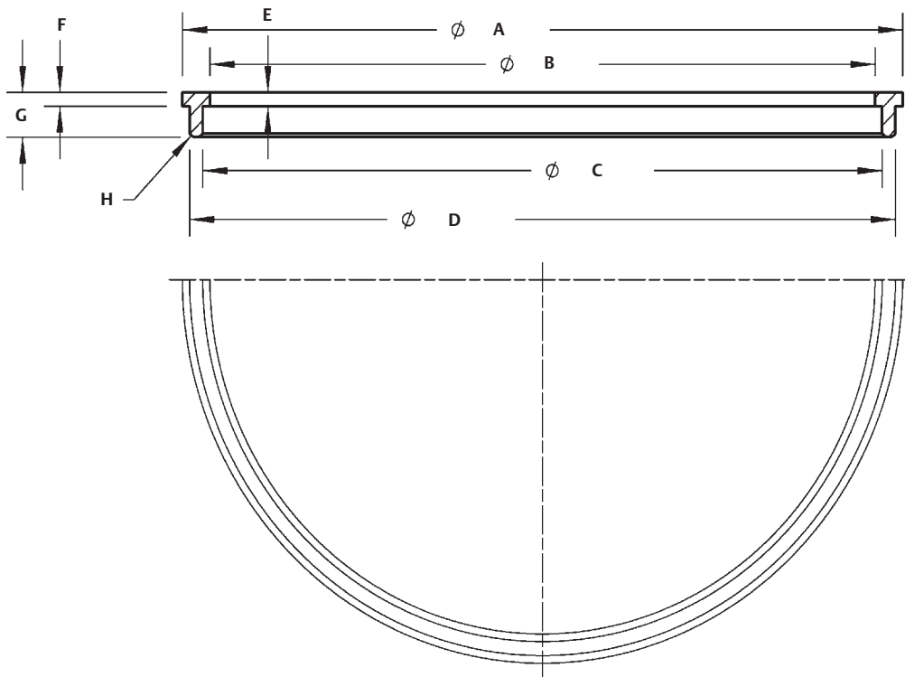
Figure 6. Outil d'installation du clapet Bore Seal
