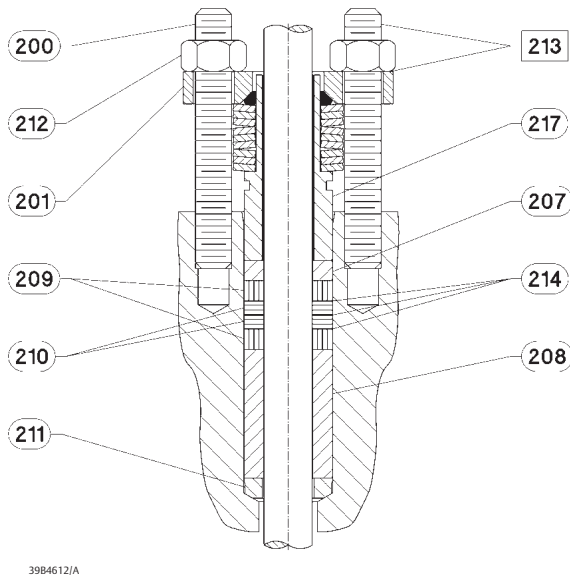
Garniture type ENVIRO-SEAL avec garniture graphite ULF
