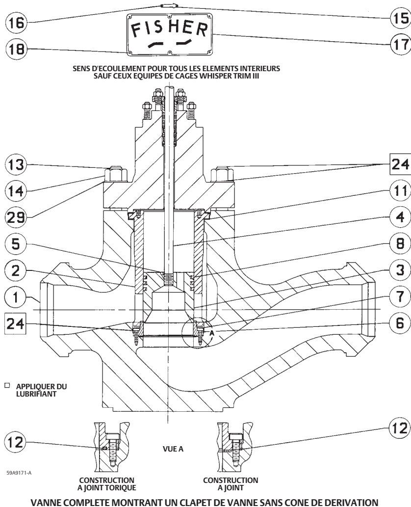
Figure 12. Vanne EHD de Fisher
