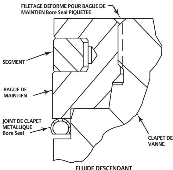
Figure 7. Piquetage des filetages de bague de maintien Bore Seal
