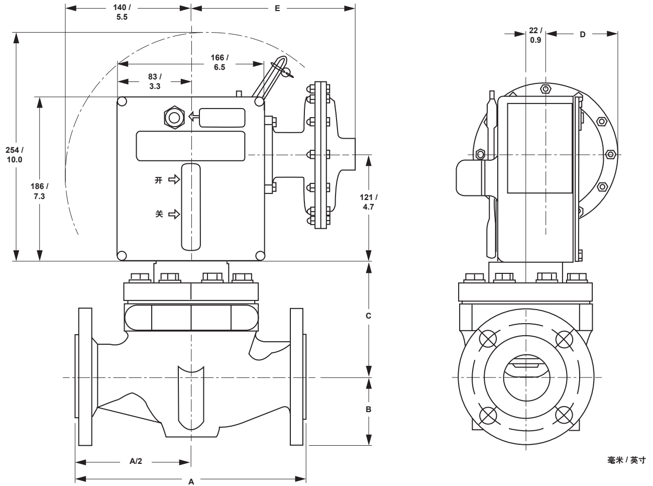
图 6. 配有脱扣机构 (BM) 和压力传感器 (BMS) 的 FEQ 型切断阀
