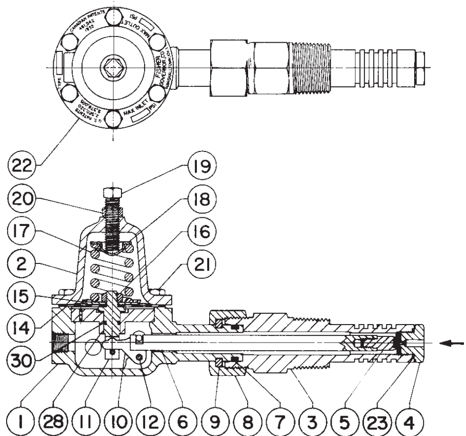
Figure 1. Détendeur série 1305
