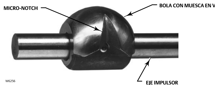
Figura 15. Eje impulsor de metal típico de esfera Micro-Notch
