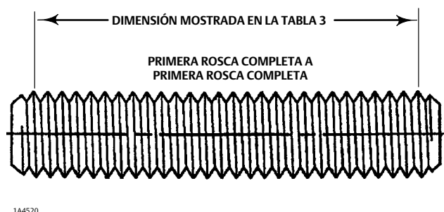
Figura 2. Longitud del espárrago de la brida para extremo protector del sello
