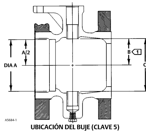
Figure 28. Ubicación del buje
