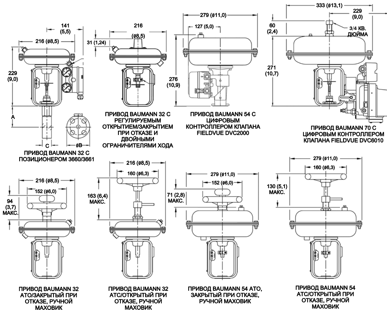
Рис. 10. Габаритные чертежи
