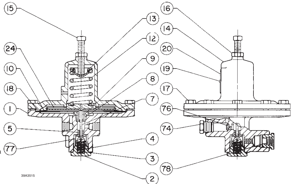
Figura 2. Conjunto del Tipo 6492L
