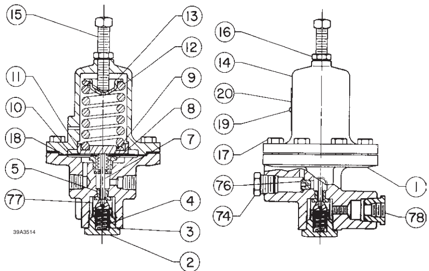
Figura 1. Conjunto del Tipo 6492H
