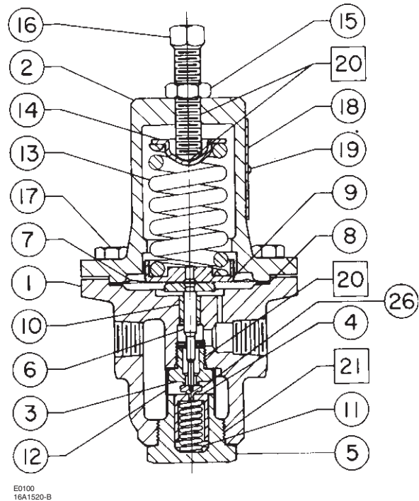
Figuur 1: Stuurdrukregelaar type 6392
