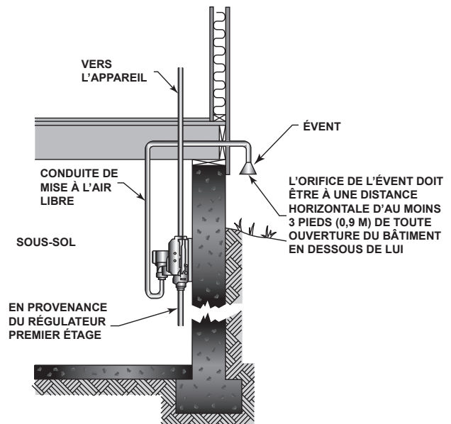
Figure 4. Installation dans un sous-sol
