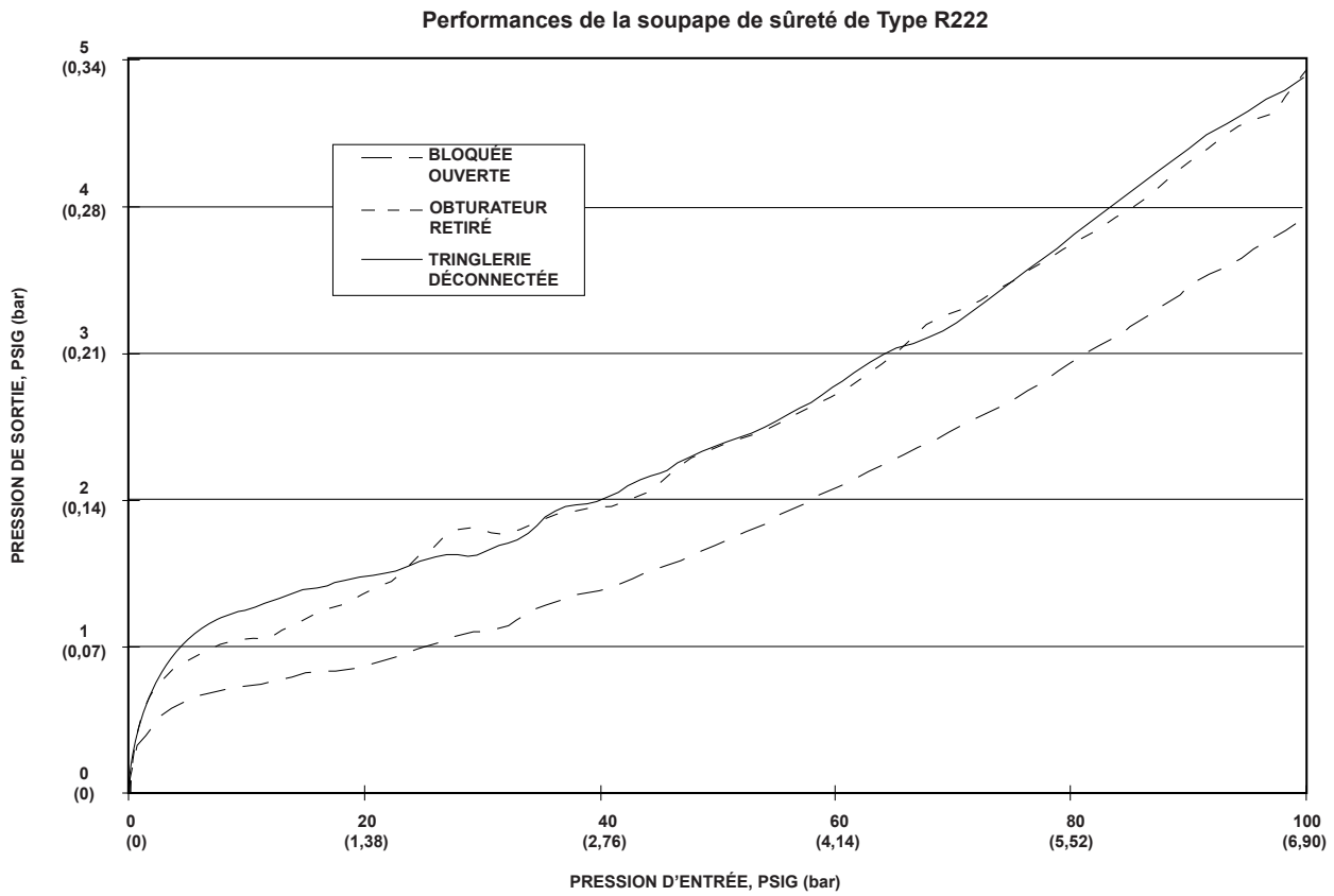
Figure 6. Courbes de la Soupape de Sûreté Pour le R122H et le R222 (suite)
