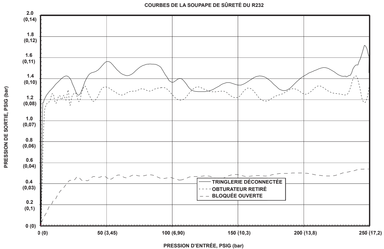
Figure 6. Courbes de la Soupape de Sûreté Pour le R232
