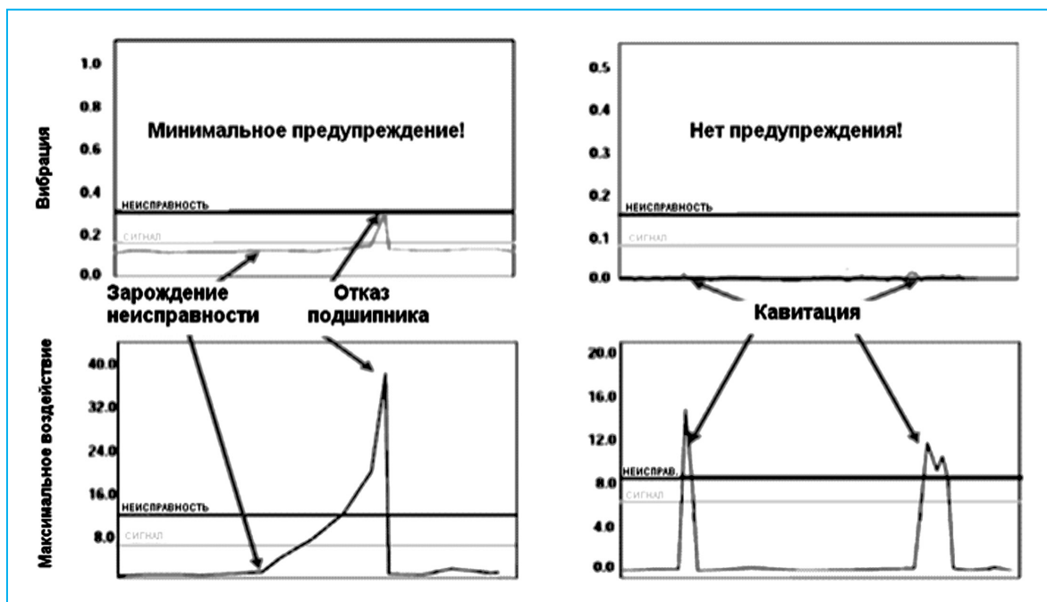
Рис. 2. Что значит определение максимального воздействия? На рисунке показан уровень суммарной вибрации и значение PeakVue. Значение максимума определяется с помощью быстродействующих измерительных устройств при 50000 наборов данных в секунду. Измерение PeakVue позволяет определить микровзрыв, происходящий при соударении металла внутри установки. PeakVue представляет собой максимальное значение такого соударения
