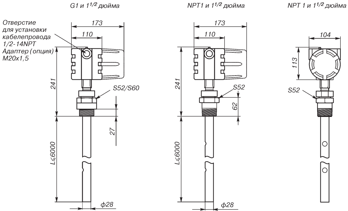
Резьбовое присоединение.
