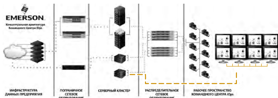
Рис. 1. Архитектура командного центра интегрированных операций
