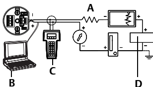
644 hovedmonteret transmitter
