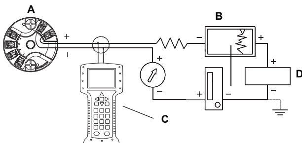
Slika 1. Spajanje uređaja za komunikaciju na petlju laboratorija
