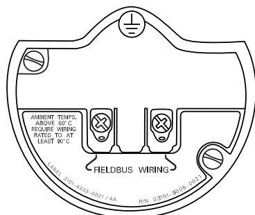
Figur 1. Fieldbus-rekkeklemme
