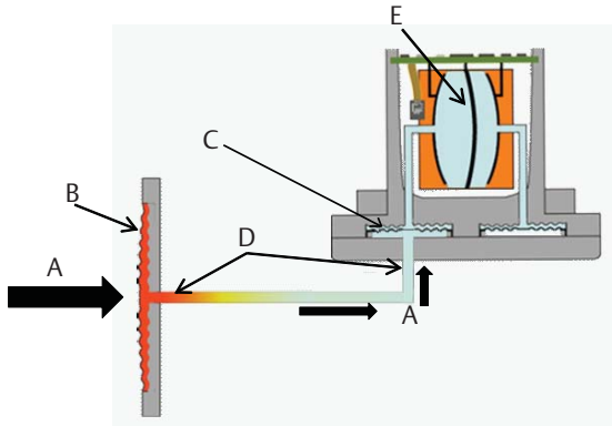
Figura 1. Percurso da pressão num Sistema de Vedação do Nível DP Standard
