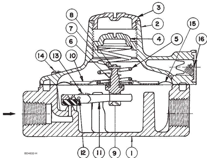
Afbeelding 1. 912 serie drukregelaar
