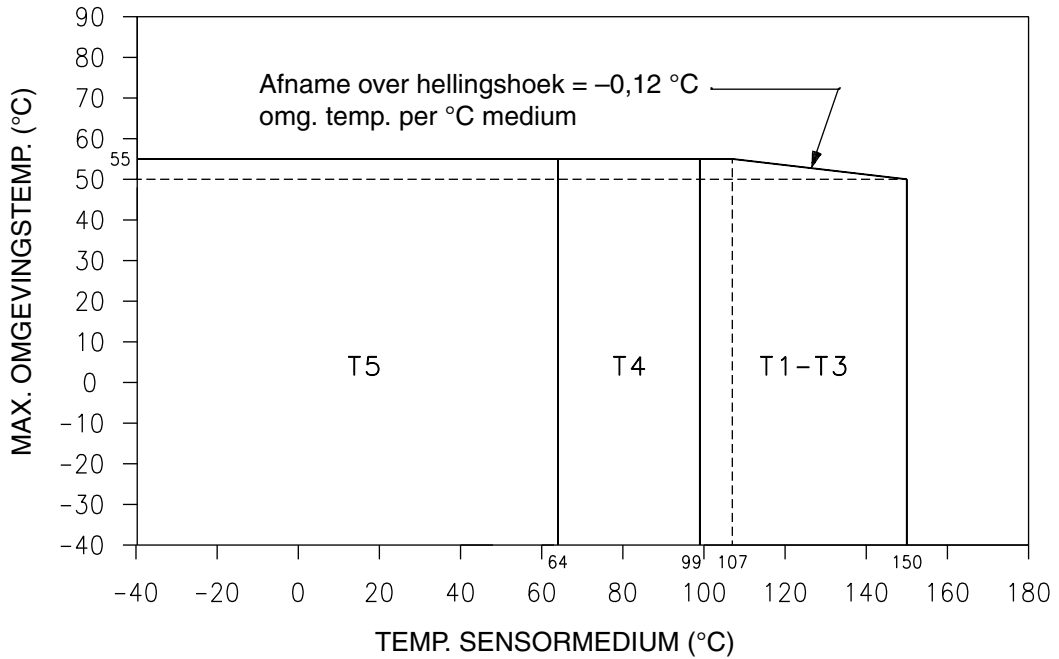
VOLGENS ATEX TOEGESTANE TEMP.KLASSE VAN F-SERIE SENSOR MET INTEGRAAL GEMONTEERDE KERNPROCESSOR OP BASIS VAN TEMP. OMGEVING/MEDIUM
