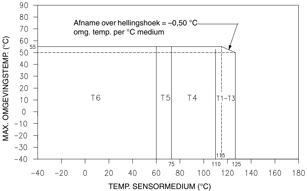
VOLGENS ATEX TOEGESTANE TEMP.KLASSE VAN F-SERIE SENSOR MET INTEGRAAL GEMONTEERDE IFT9701 OP BASIS VAN TEMP. OMGEVING/MEDIUM
