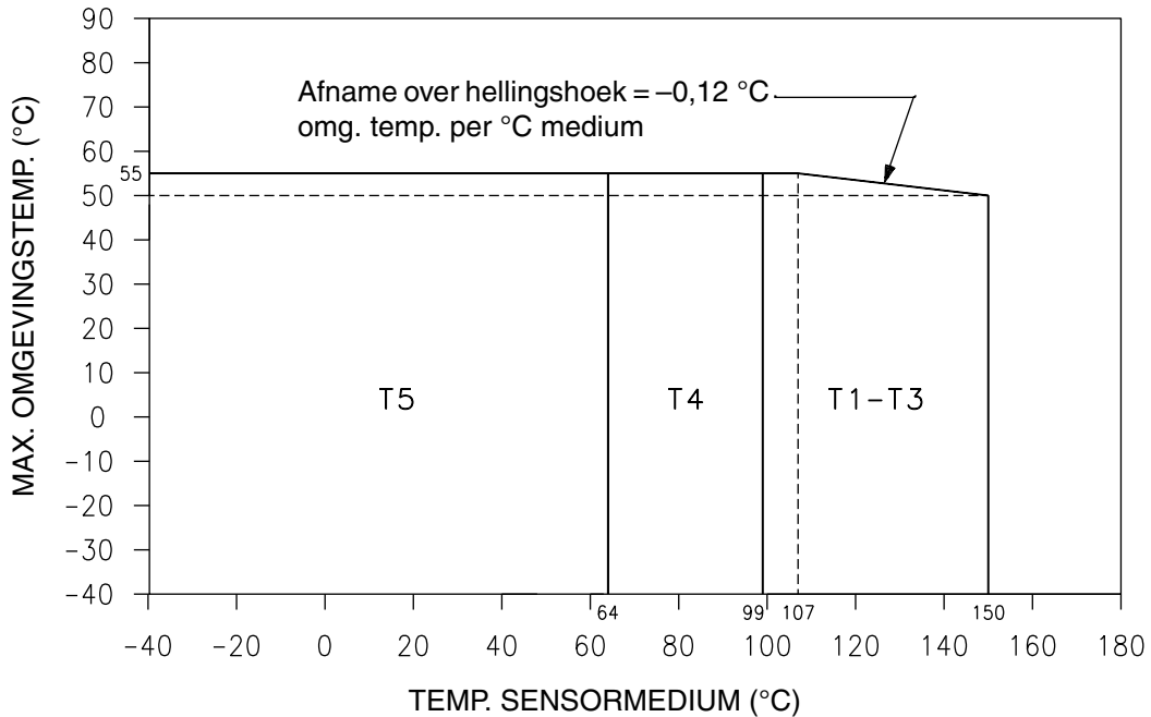
VOLGENS ATEX TOEGESTANE TEMP. KLASSE VAN F-SERIE SENSOR MET INTEGRAAL GEMONTEERDE MODEL 1700/2700 TRANSMITTER OP BASIS VAN TEMP. OMGEVING/MEDIUM
