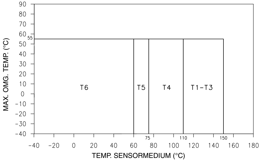
VOLGENS ATEX TOEGESTANE TEMP.KLASSE VAN F-SERIE SENSOR MET INTEGRALE AANSLUITDOOS OP BASIS VAN TEMP. OMGEVING/MEDIUM
