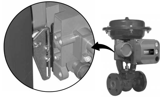
SYSTEME DE CONTRE- REACTION SANS LIAISON
