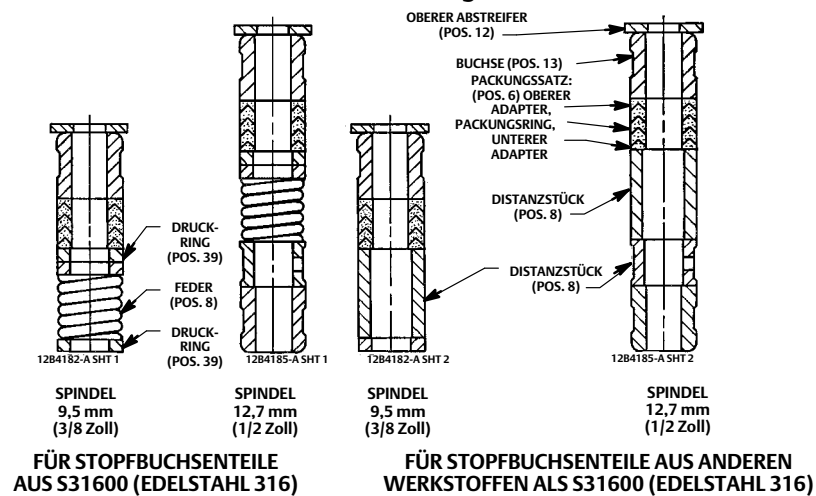
Abbildung 8. PTFE-Packung für den Einsatz in ENVIRO-SEAL Faltenbalg-Oberteilen
