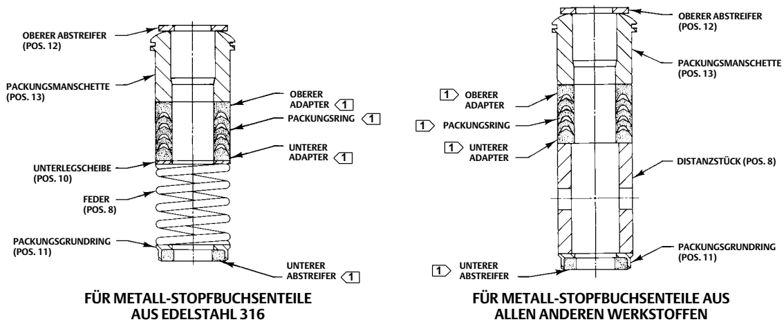
Abbildung 3. PTFE-Dachmanschettenpackungen für Standard- und verlängertes Oberteil
