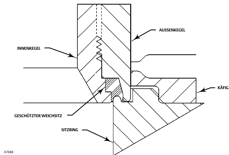
Abbildung 6. TSO (dicht schließend), Detail des geschützten Weichsitzes
