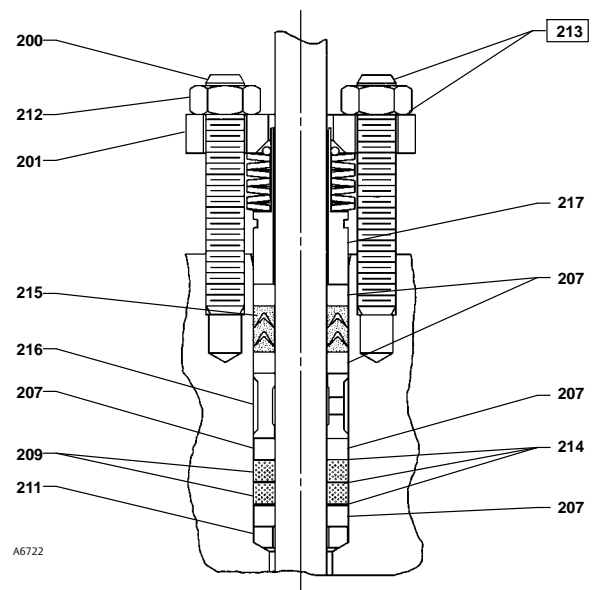
Abbildung 13. Typisches ENVIRO-SEAL Packungssystem mit Duplexpackung
