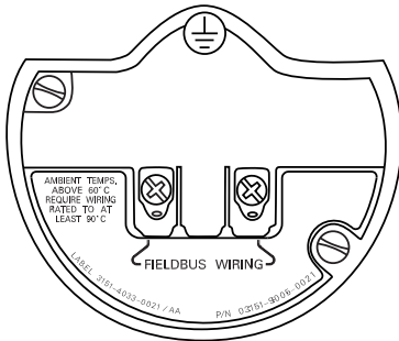
Figura 1. Bloco de terminais Fieldbus
