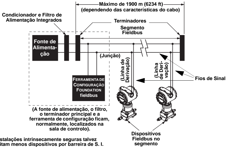
Figura 2. Ligação de fios no campo do indicador FOUNDATION fieldbus
