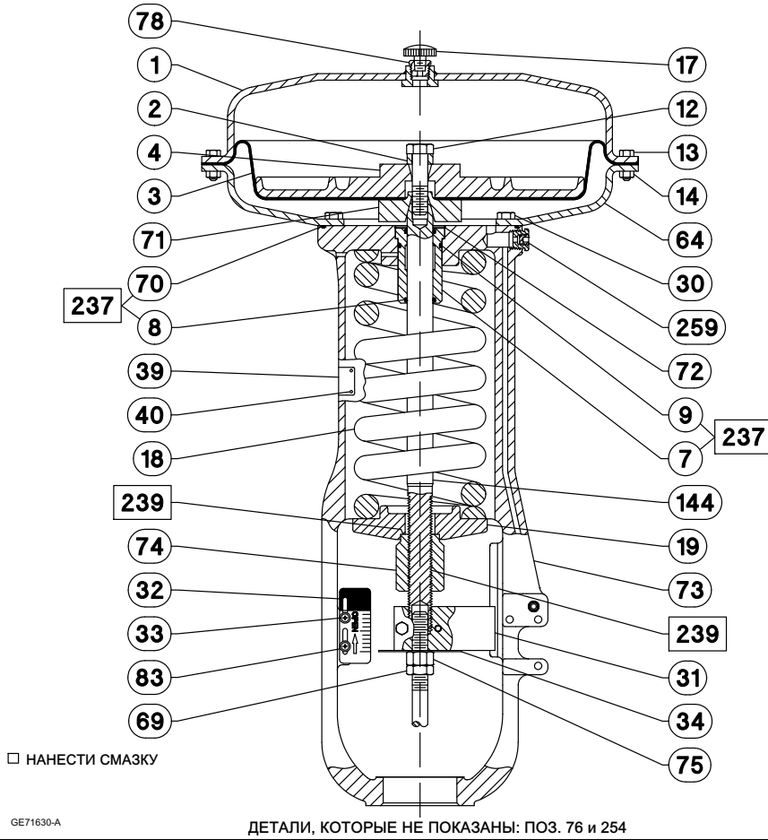
Рис. 9. Привод Fisher модели 667 размером 70i и 76i
