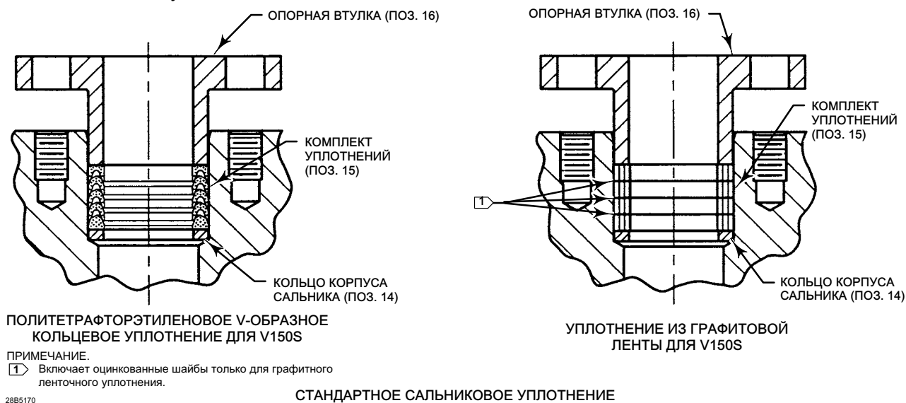
Рис. 6. Компоновки уплотнений
