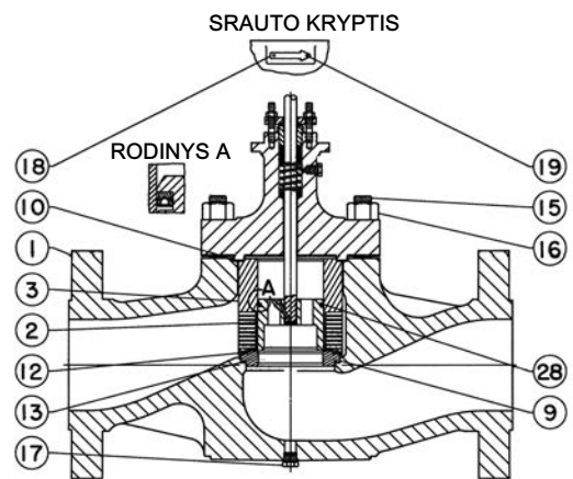
NPS 8 x 6 CL900 VOŽTUVO TARPIKLIŲ SU PASIRINKTINIŲ IŠLEIDIMO KAIŠČIU DUOMENYS
