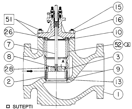
NPS 12 x 8 VOŽTUVAS
