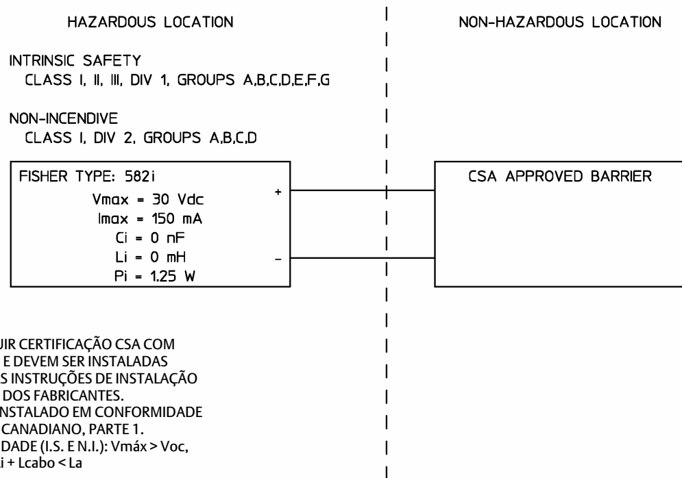
Figura 28. Diagrama do Circuito CSA para o Conversor 582i da Fisher (Esquema de Instalação GE28591)
