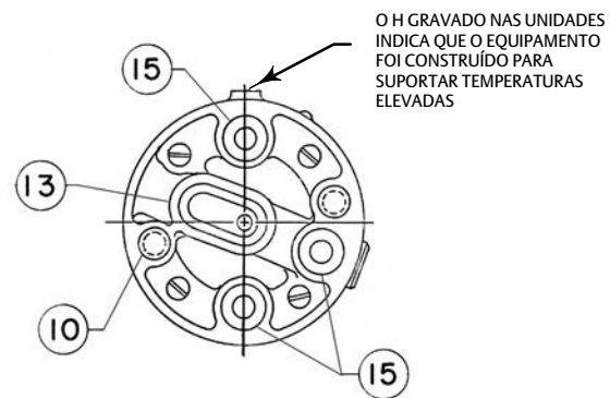
Figura 23. Relé 83L
