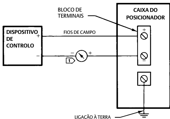
Figura 9. Diagrama de Fios de Campo Típico
