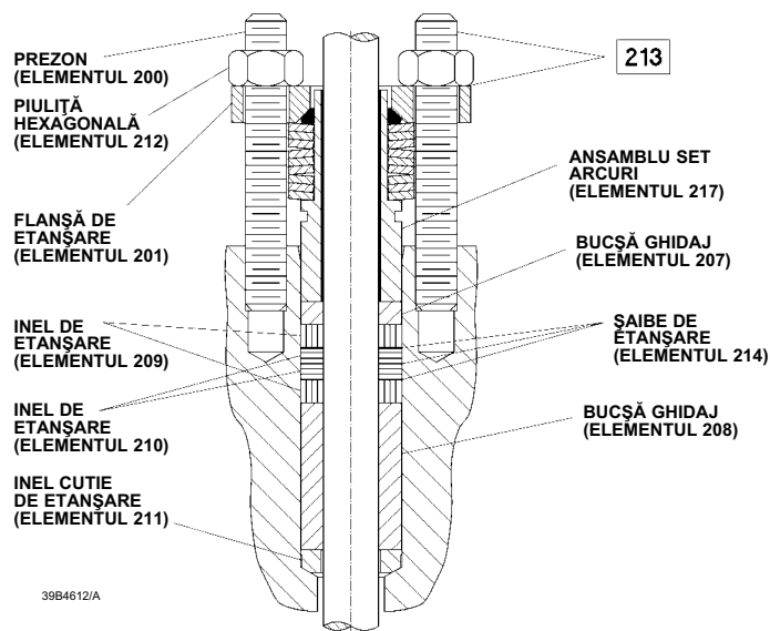
Sistem tipic ENVIRO-SEAL de etanșare cu garnitură ULF din grafit
