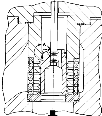
FLUX DISPOZITIV DE ECHILIBRARE NPS 3 - 6 HPT CU LOCAȘ CAVITOL III CU 3 TREPTE
