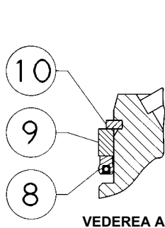
FLUX DISPOZITIV DE ECHILIBRARE NPS 2 HPS CU LOCAȘ CAVITOL III CU 3 TREPTE
