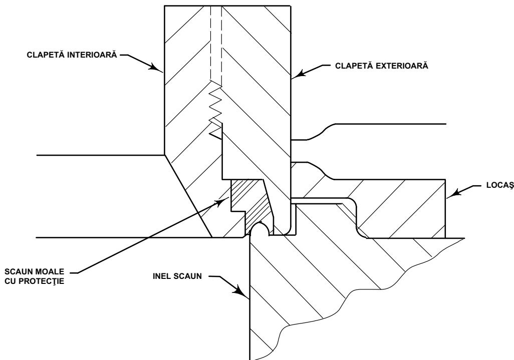
Figura 6. Detaliu scaun moale cu protecție
