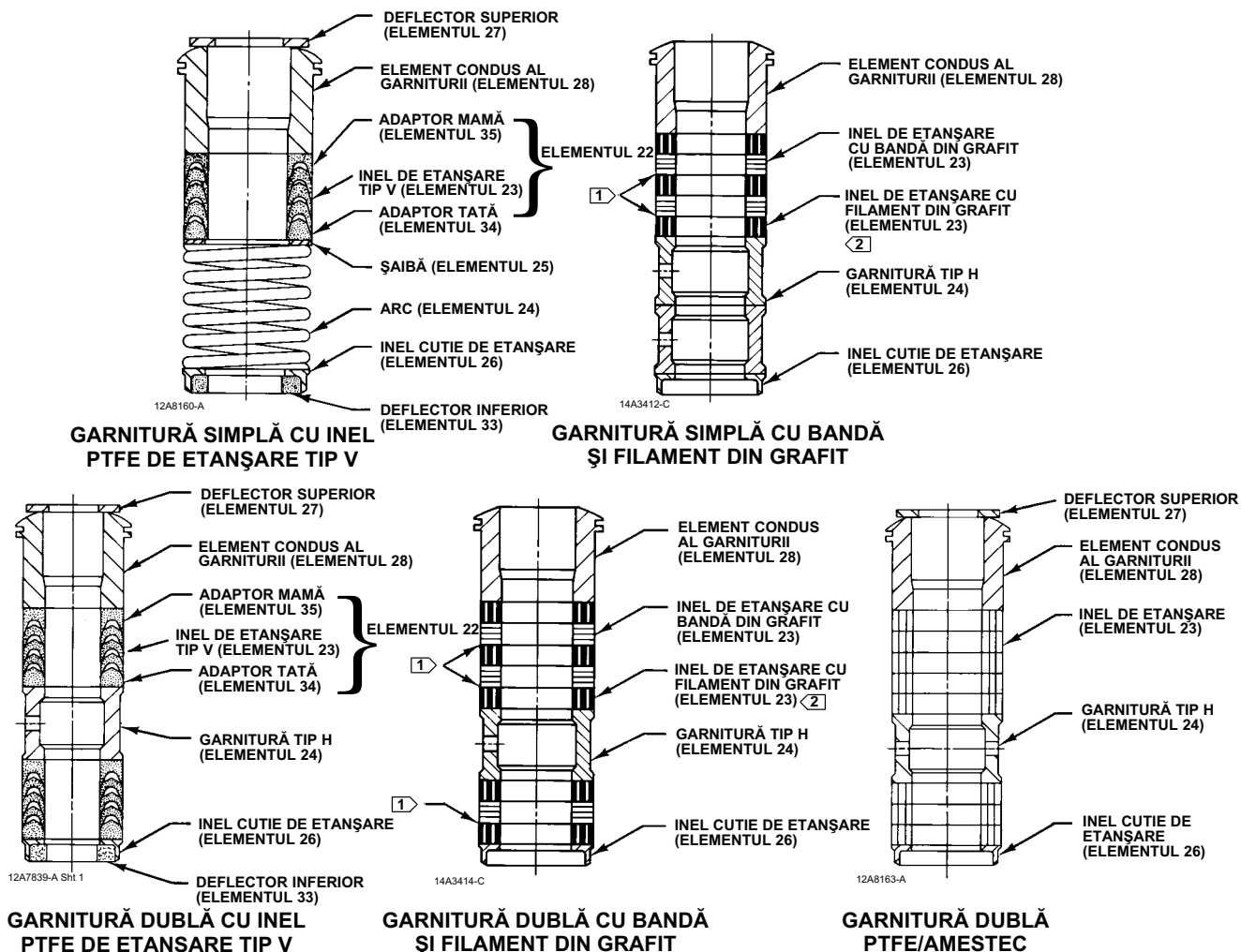
Figura 3. Configurațiile garniturii
