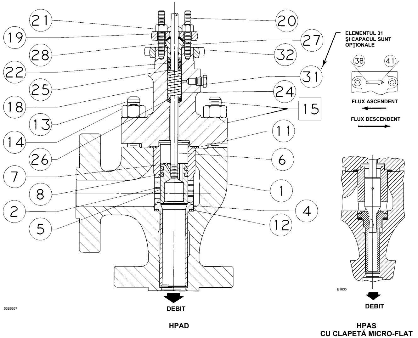
Figura 18. Supapă NPS 2 HPAD
