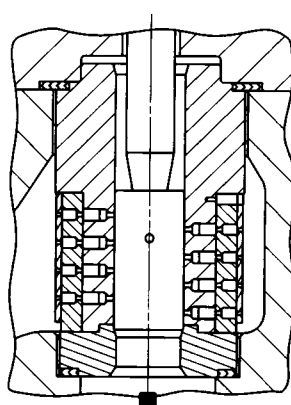
FLUX DISPOZITIV DE ECHILIBRARE NPS 2 HPS CU LOCAȘ CAVITOL III CU 3 TREPTE
