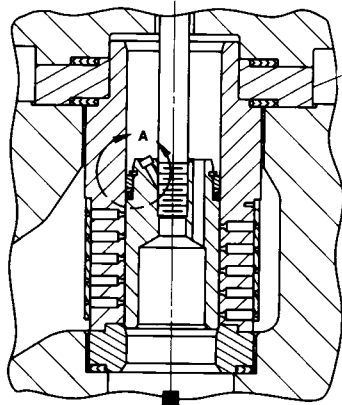
FLUX DISPOZITIV DE ECHILIBRARE NPS 2 HPT CU LOCAȘ CAVITOL III CU 2 TREPTE
