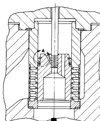
FLUX DISPOZITIV DE ECHILIBRARE NPS 3 - 6 HPT CU LOCAȘ CAVITOL III CU 2 TREPTE
