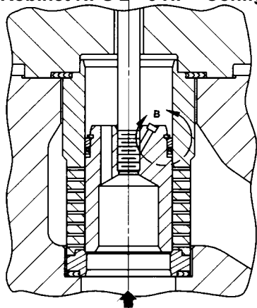
FLUX DISPOZITIV DE ECHILIBRARE HPT, HPAT CU LOCAȘ WHISPER III, DISPONIBIL ÎN HPD, HPAD, HPS ȘI HPAS (NPS 2)
