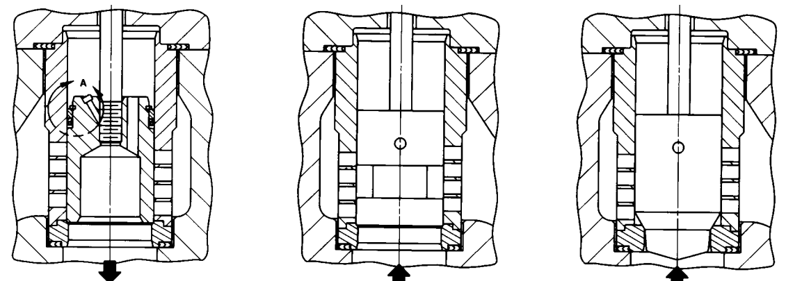
FLUX DISPOZITIV DE ECHILIBRARE HPT, HPAT (TOATE DIMENSIUNILE)
