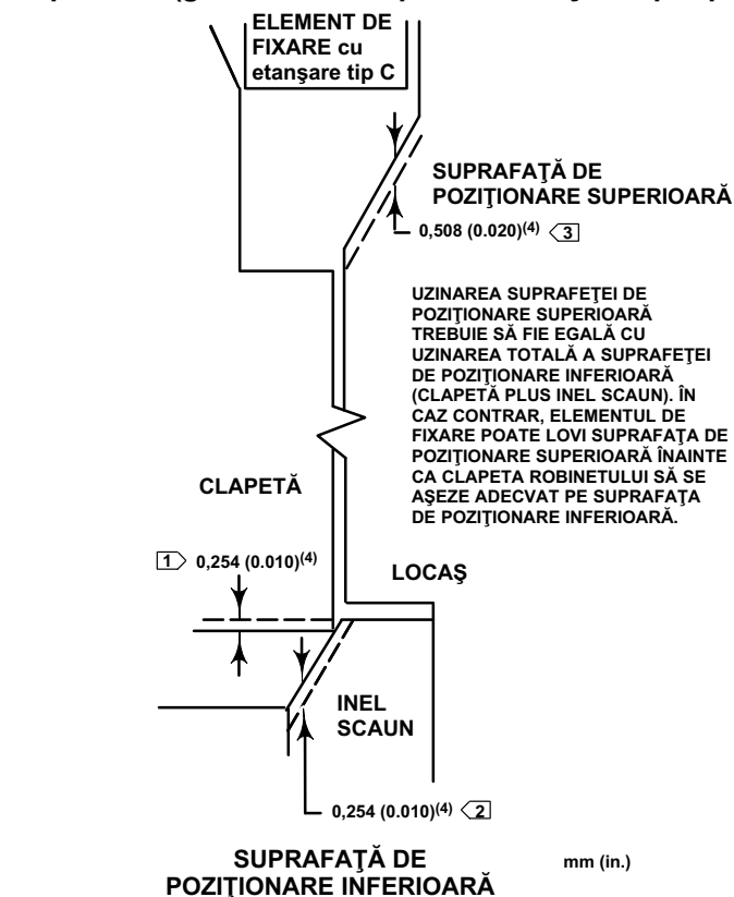
Figura 16. Exemplu de uzinare a suprafețelor de poziționare inferioare (clapetă robinet pe inel scaun) și superioare (garnitură de clapetă cu etanșare tip C pe locaș)
