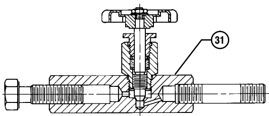
ROBINET DE LUBRIFIERE/IZOLARE
