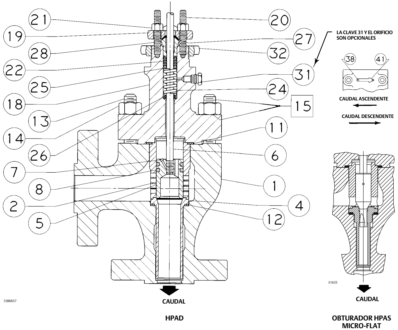
Figura 18. Válvula NPS 2 HPAD
