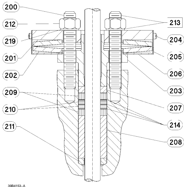
Sistema de empaque de grafito ULF HIGH-SEAL típico
