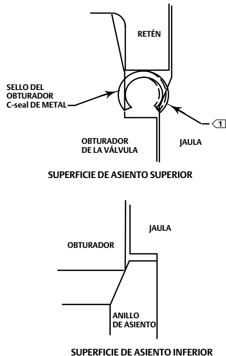
Figura 15. Superficies de asiento inferior (obturador de la válvula al anillo de asiento) y superior (sello del obturador C-seal a la jaula)
