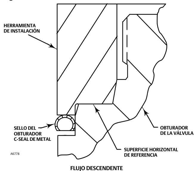
Figura 13. Instalación del sello del obturador C-seal usando la herramienta de instalación
