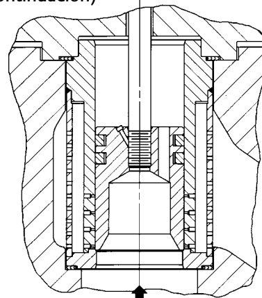
FLUJO WHISPER III NIVEL D DEL INTERNO DE HPD DE NPS 4
