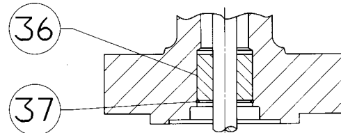
CONJUNTO DE DEFLECTOR DEL BONETE DE LA EXTENSIÓN (SOLO NPS 2) (ESFÉRICO Y DE ÁNGULO)
