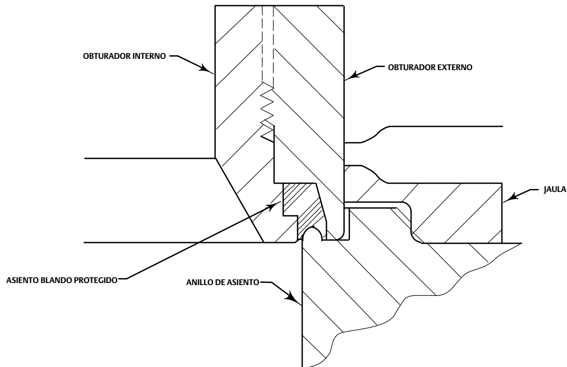
Figura 6. Detalle del asiento blando protegido
