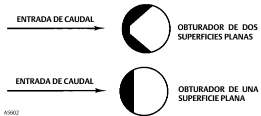
ORIENTACIÓN DEL OBTURADOR DE LA VÁLVULA MICRO-FLAT
