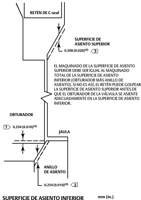
Figura 16. Ejemplo de maquinado de las superficies de asiento inferior (obturador de la válvula al anillo de asiento) y superior (sello del obturador C-seal a la Jaula)
