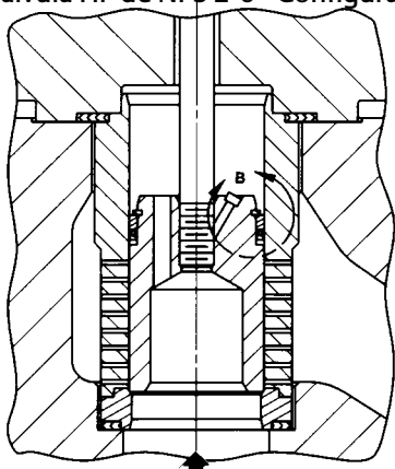
FLUJO INTERNOS HPT, HPA, HPS, HPS III, DISPONIBLES SOLO EN HPD, HPAD, HPS Y HPAS (NPS 2)
