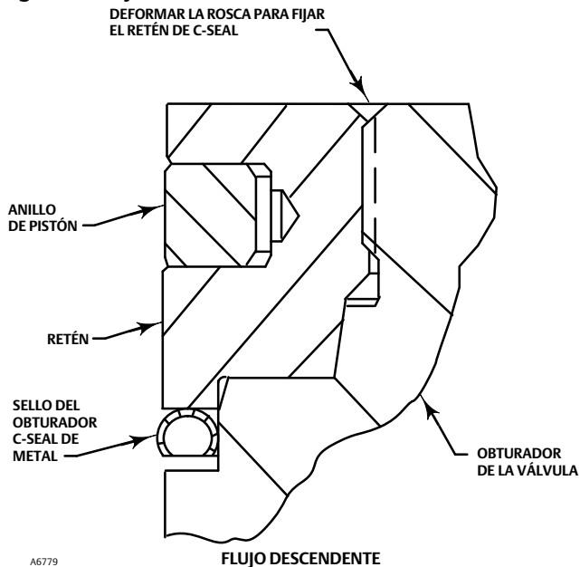
Figura 14. Fijar las roscas del retén de C-seal
