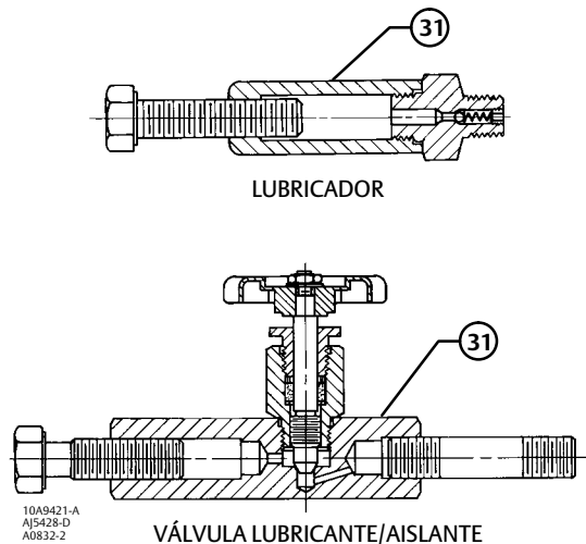
Figura 2. Lubricador y válvula lubricante/aislante
