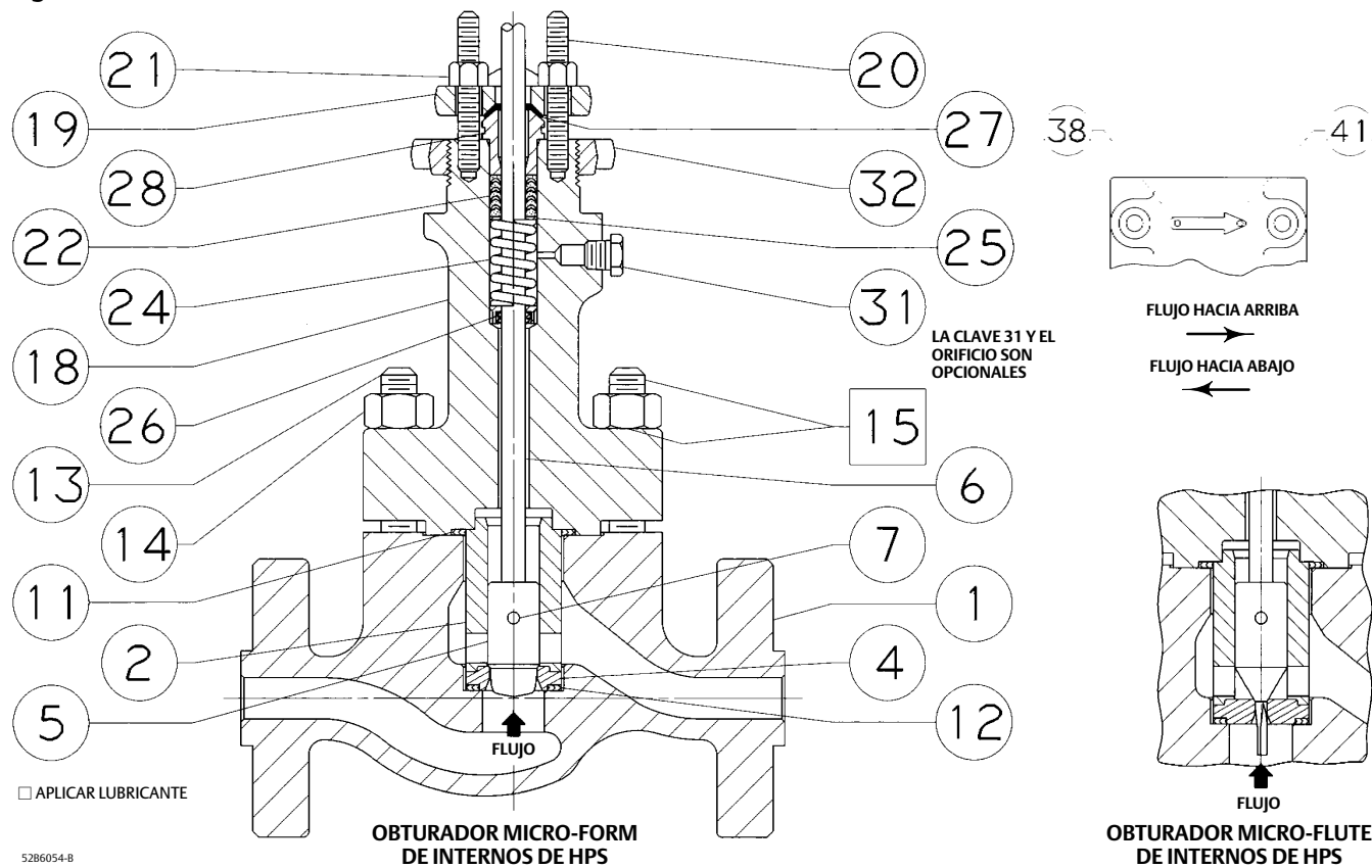
Figura 17. Válvula HPS de NPS 1
