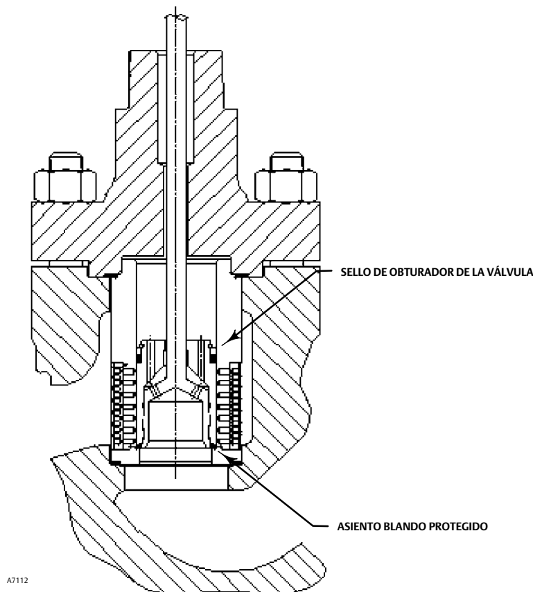
Figura 8. Internos TSO equilibrados típicos (diámetro de puerto de 1,6875 pulgadas)
