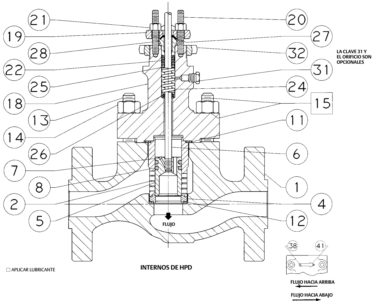
Figura 19. Válvula HPD de NPS 2-6
