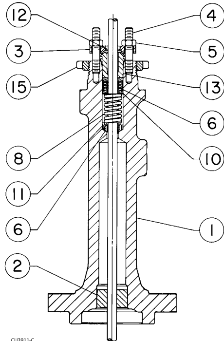
COBERTURA DE PROLONGAMENTO TIPO 1 OU 2
