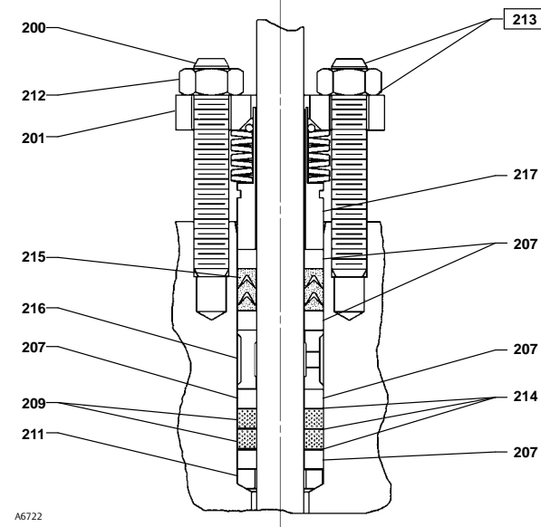
Figura 20. Sistema de Empanque Típico ENVIRO-SEAL com Empanque Duplex da Fisher
