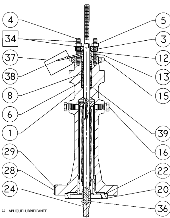
COBERTURA DE VEDAÇÃO DE FOLES ENVIRO-SEAL
