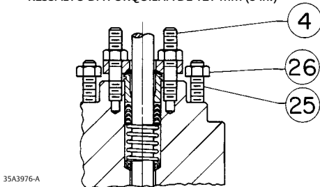
DETALHE DOS PARAFUSOS DO RESSALTO DA FORQUILHA DE NPS 12 x 8 CL900
