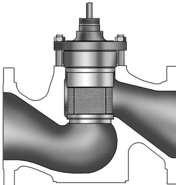
Figura 2. Vista em Corte dos Internos de WhisperFlo da Fisher, Corpo de Válvula Típico
