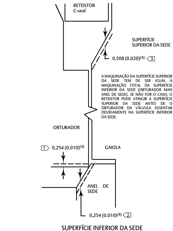
Figura 14. Exemplo de Maquinação das Superfícies Inferior (Obturador da Válvula para Anel de Sede) e Superior (Vedação do Obturador C-seal para a Gaiola) da Sede
