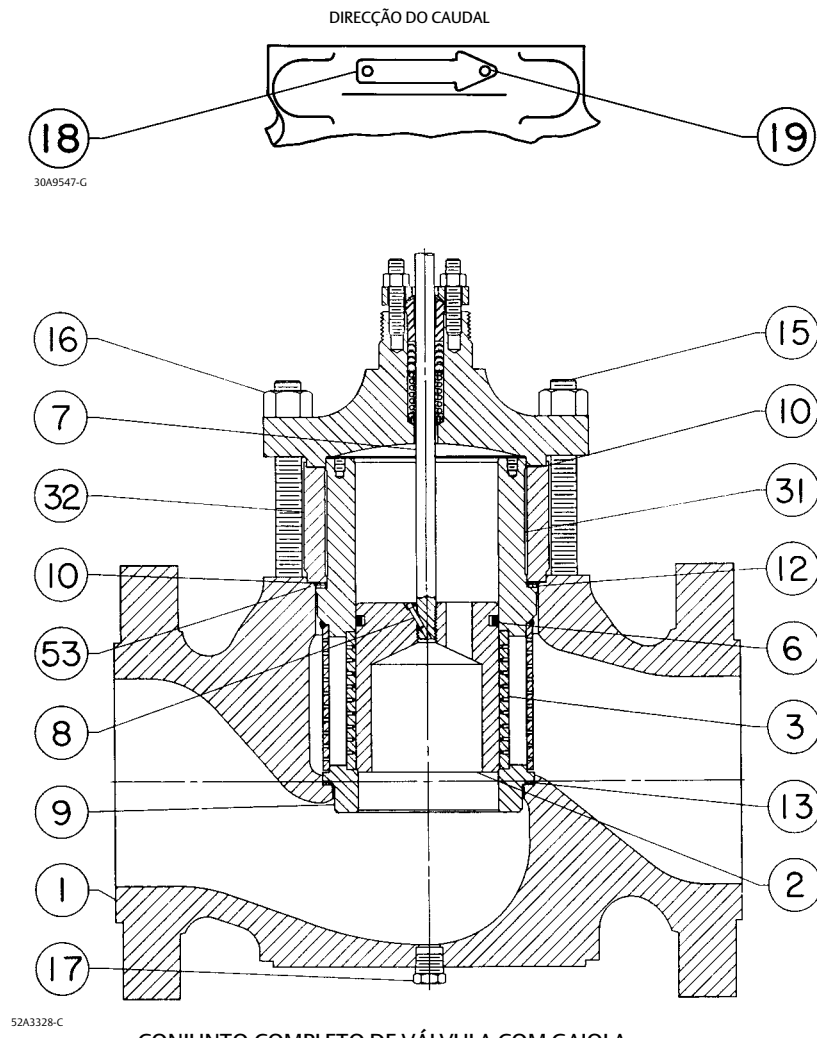
CONJUNTO COMPLETO DE VÁLVULA COM GAIOLA WHISPER TRIM III, ANEL DO PISTÃO DE GRAFITE INDIVIDUAL E BUJÃO DE DRENAGEM OPCIONAL
