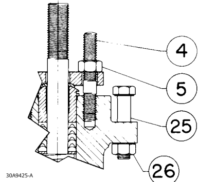
DETALHE DOS PARAFUSOS DO ACTUADOR NO RESSALTO DA FORQUILHA DE 127 mm (5 in.)
