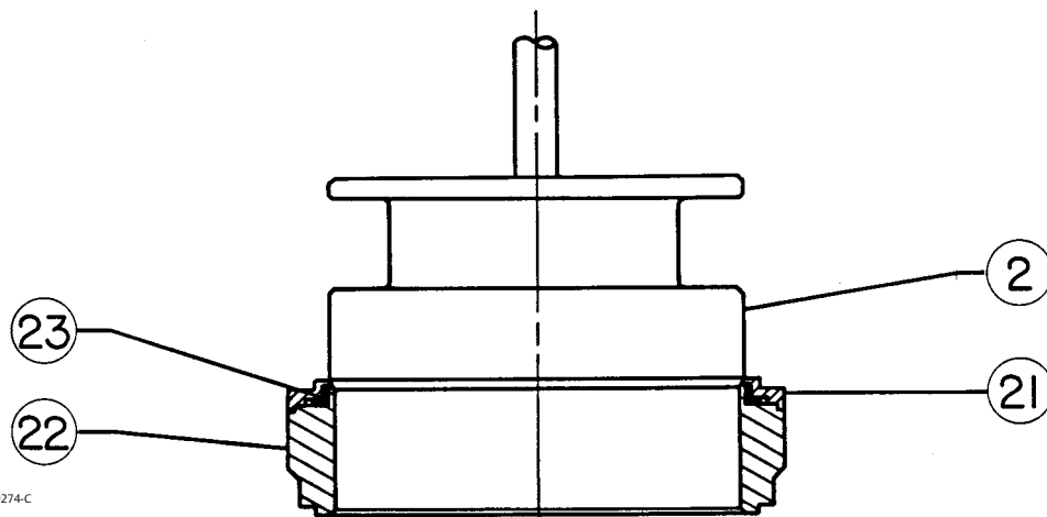
DETALHE DA SEDE DE ELASTÓMERO
