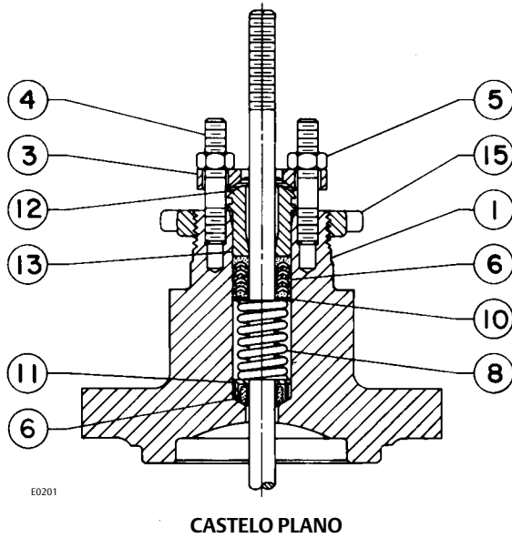
Figura 21. Castelo Fisher típico com conjunto de juntas de anel V de PTFE simples
