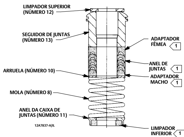
Figura 4. Disposições das juntas de PTFE de anel V
