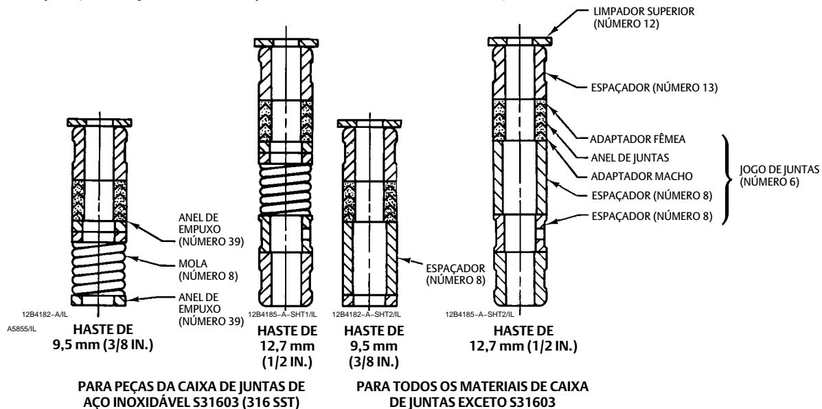
Figura 15. Disposição das juntas de PTFE para Uso com Castelos de Vedação de folios Fisher ENVIRO-SEAL
