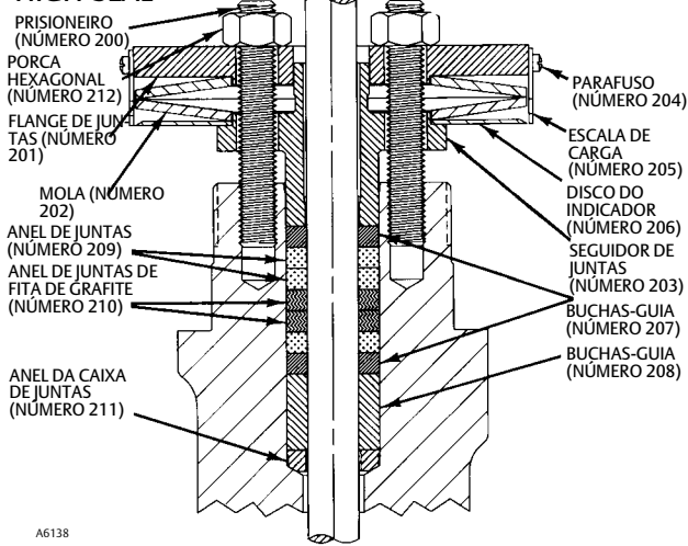
Figura 17. Sistema típico de juntas Fisher HIGH-SEAL
