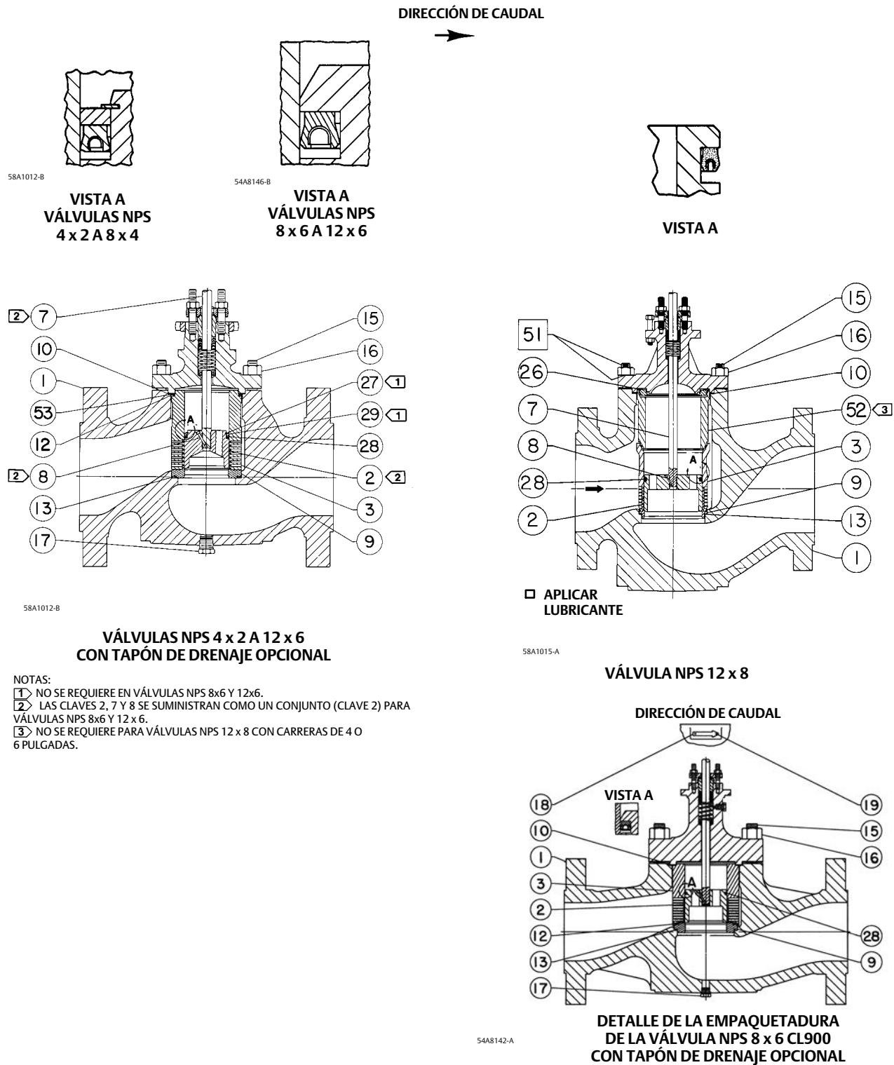
Figura 26. Válvula Fisher NPS 4x2 a 12x8 con jaula Cavitrol III de una etapa
