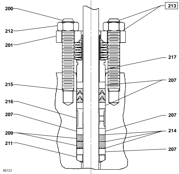
Figura 20. Sistema típico de empaque Fisher ENVIRO-SEAL con empaque dúplex
