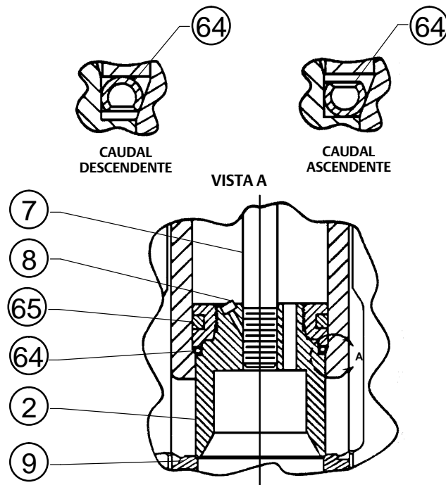
Figura 9. Fisher EWD con internos C-seal
