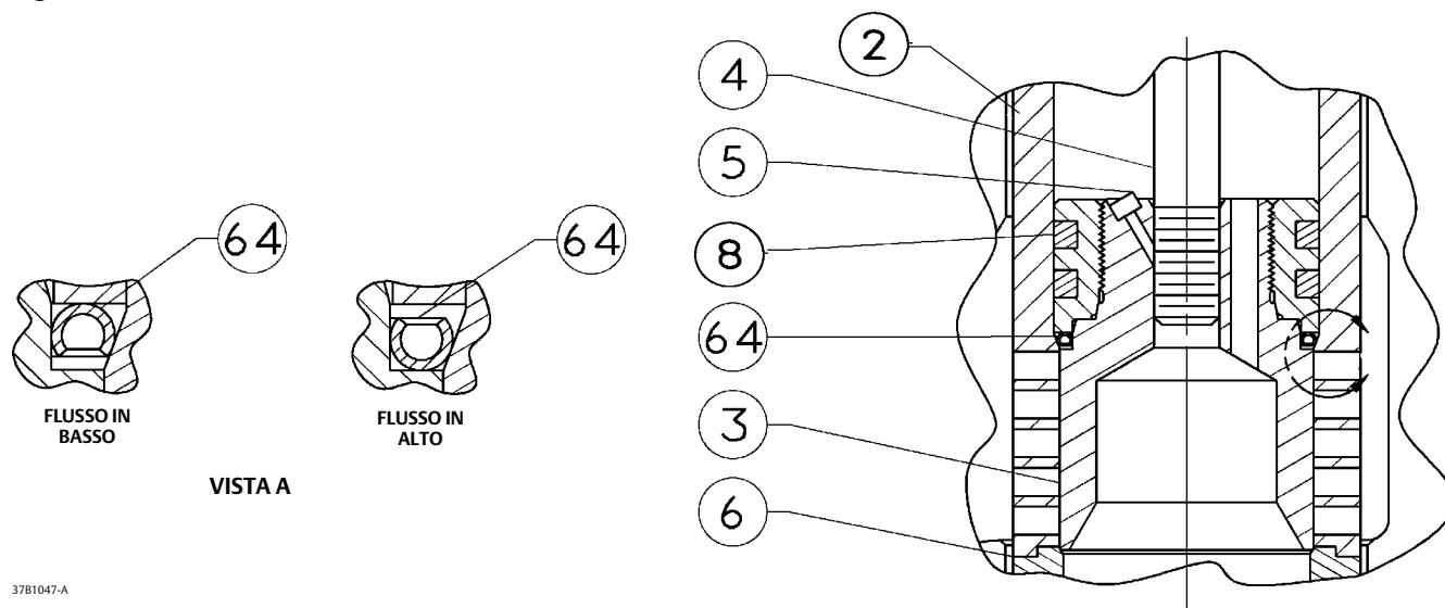
Figura 10. Valvola EHD Fisher con trim C-seal
