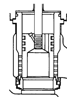
57A2887-A DETTAGLIO DELLA GABBIA WHISPER TRIM III PER CORPI VALVOLA DA 3 A 4 POLLICI
