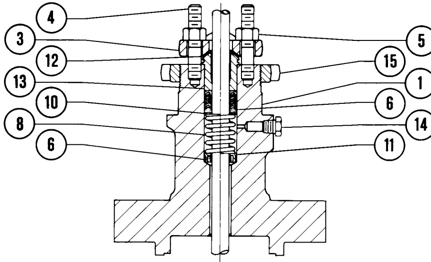
CAPPELLO CON RISALTO DELLA STAFFA DA 71 mm (2-3/16 IN.) CON BADERNA IN PTFE SINGOLA
