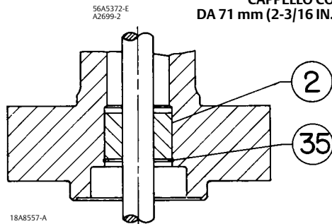
DETTAGLIO DEL DEFLETTORE E DELL'ANELLO DI TENUTA USATI NEL CAPPELLO ESTESO
