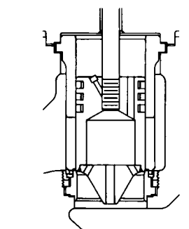
59A9166-A DETTAGLIO DELL'OTTURATORE CON CONO DEFLETTORE, SOLO PER CORPO VALVOLA DA 6 POLLICI
