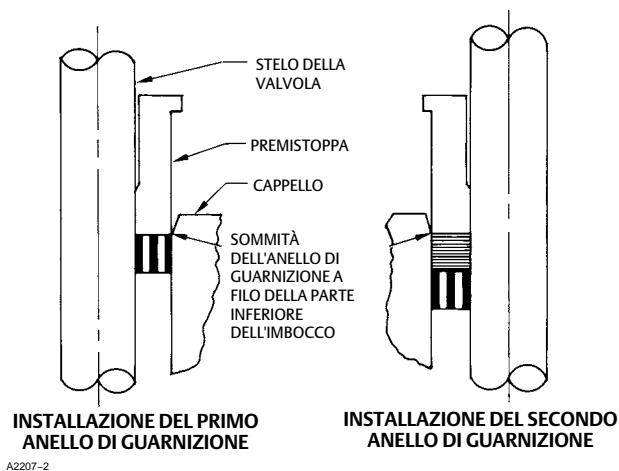
Figura 5. Installazione delle baderne a nastro e a filo di grafite una alla volta
