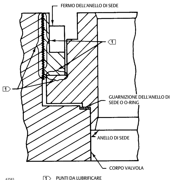
Figura 8. Superfici del trim da lubrificare
