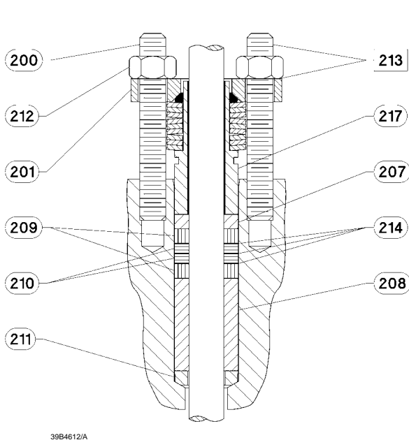
Sistema tipico di baderna ENVIRO-SEAL con baderna in grafite ULF
