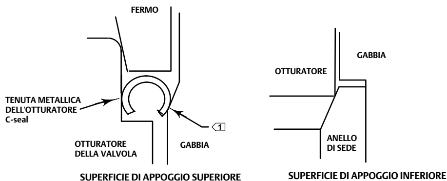
Figura 14. Superfici di appoggio inferiore (tra otturatore della valvola e anello di sede) e superiore (tra tenuta dell'otturatore C-seal e gabbia)
