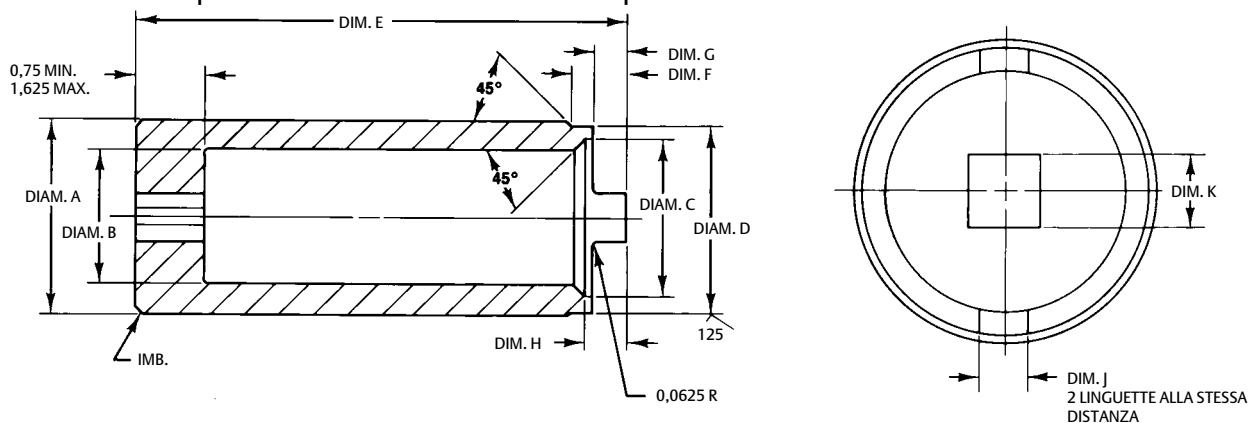
Figura 9. Informazioni per la lavorazione e l'uso dell'attrezzo per il fermo dell'anello di sede
