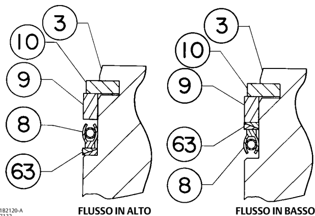
Figura 22. Valvola EHT Fisher da 3 a 6 pollici con anelli antiestrusione in PEEK
