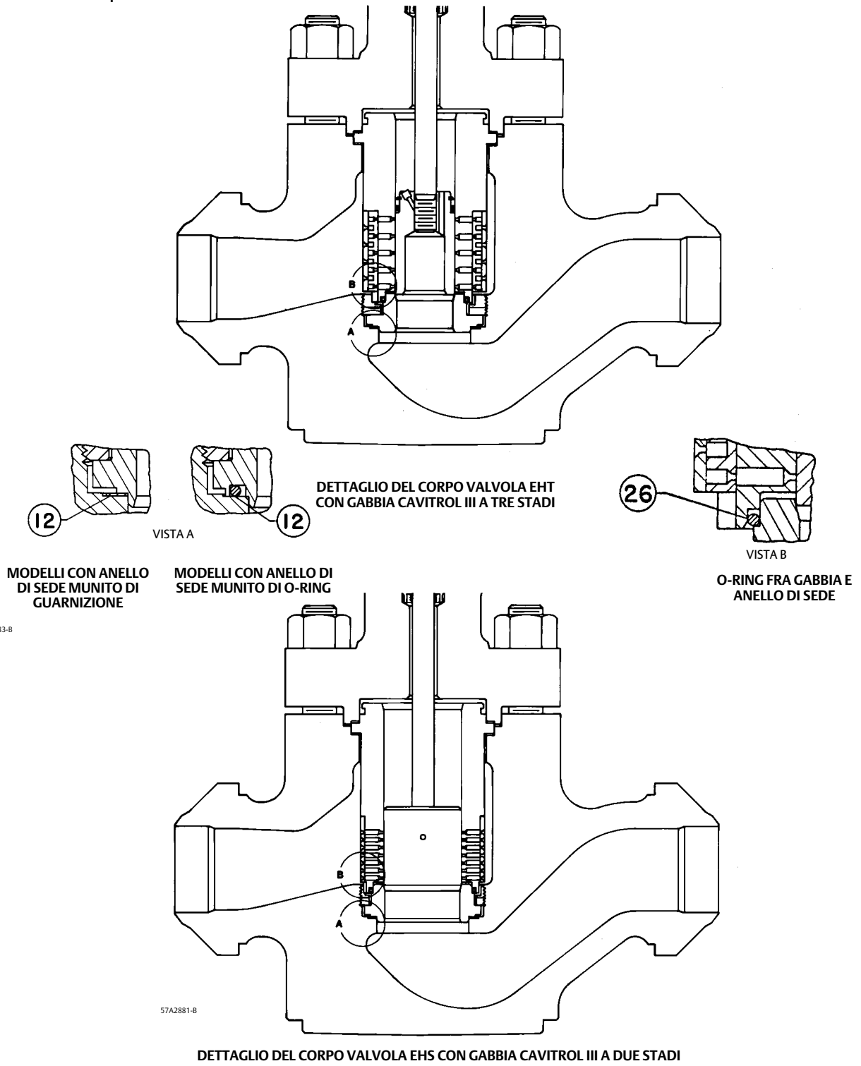
Figura 21. Modelli tipici con Cavitrol III
