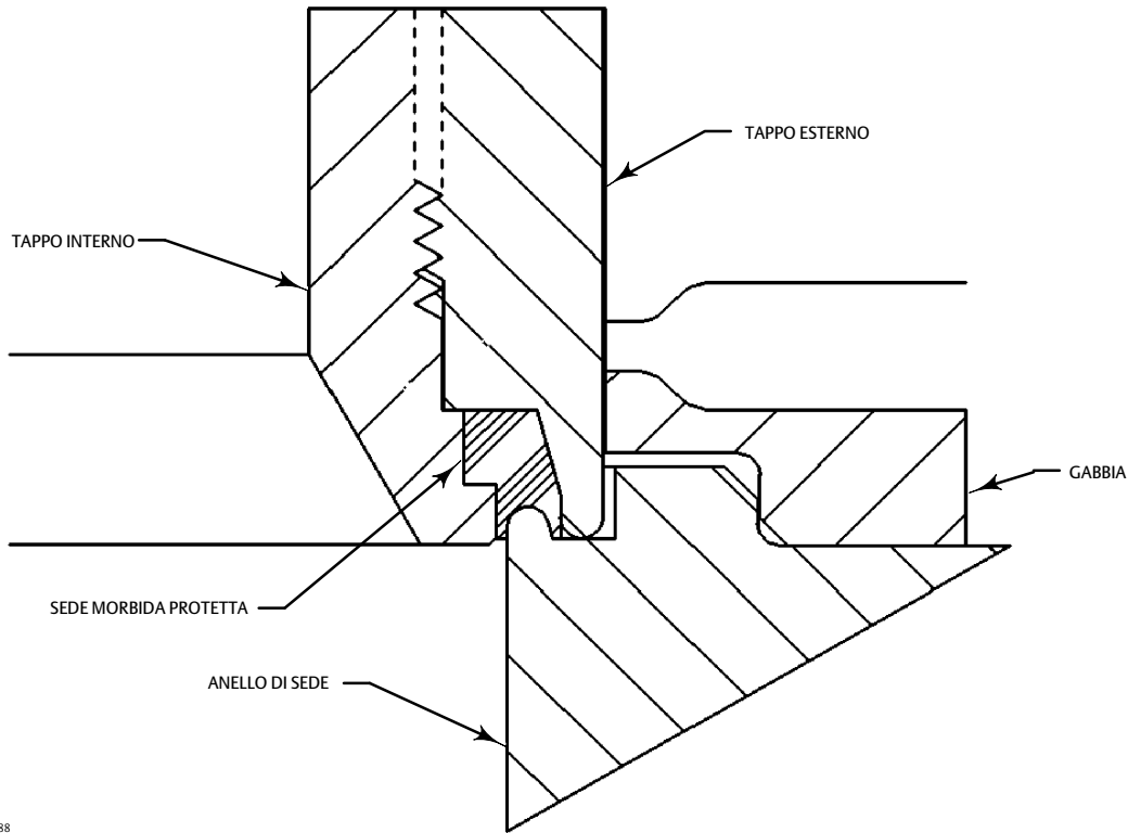
Figura 6. Dettaglio della sede morbida protetta
