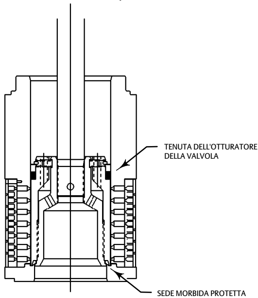
Figura 7. Trim TSO bilanciato tipico
