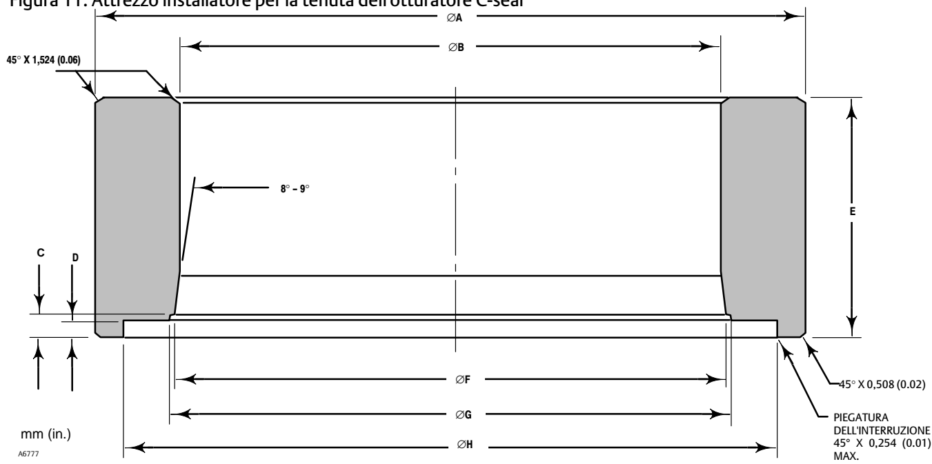
Figura 11. Attrezzo installatore per la tenuta dell'otturatore C-seal
