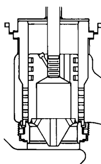
59A9188-A DETTAGLIO DELLA GABBIA WHISPER TRIM III LIVELLO A, B O C E DELL'OTTURATORE DELLA VALVOLA CON CONO DEFLETTORE, SOLO PER CORPO VALVOLA DA 6 POLLICI
