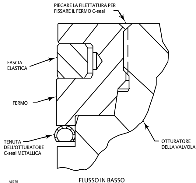
Figura 13. Piegatura delle filettature del fermo C-seal
