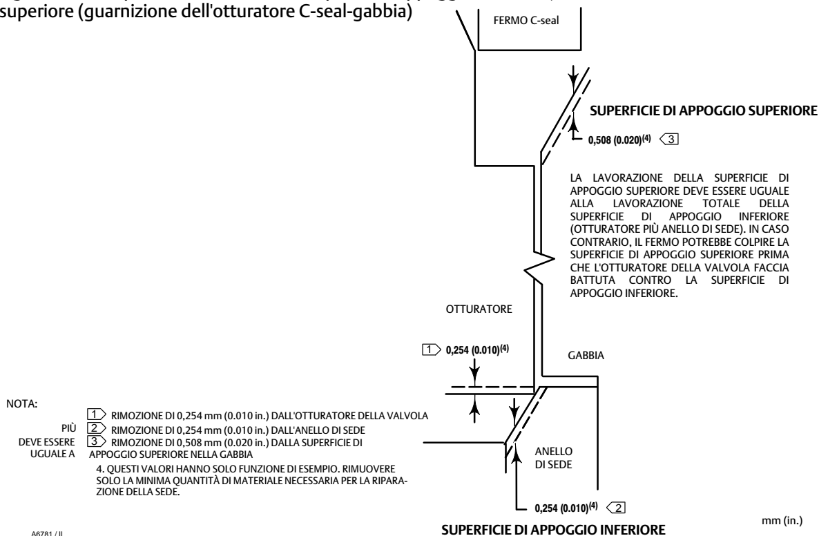
Figura 15. Esempio di lavorazione delle superfici di appoggio inferiore (otturatore della valvola-anello di sede) e superiore (guarnizione dell'otturatore C-seal-gabbia)
