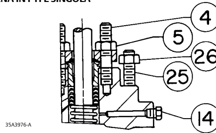
DETTAGLIO DEI BULLONI DELL'ATTUATORE CON RISALTO DELLA STAFFA DA 127 mm (5 IN.) (OPZIONALE PER I CORPI VALVOLA SERIE EH DA 3, 4 E 6 POLLICI)
