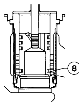
59A9190-A DETTAGLIO DELLA GABBIA WHISPER TRIM III LIVELLO D E DELL'OTTURATORE DELLA VALVOLA, SOLO PER CORPO VALVOLA DA 6 POLLICI
