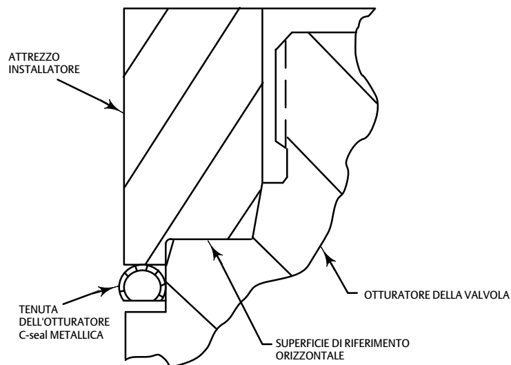
Figura 12. Installazione della guarnizione dell'otturatore C-seal con l'attrezzo installatore
