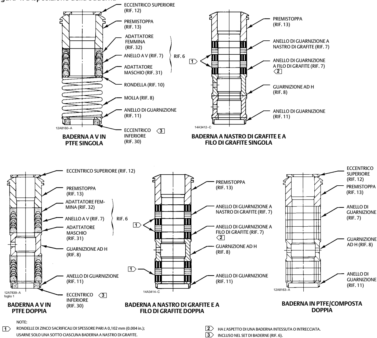
Figura 4. Disposizione della baderna
