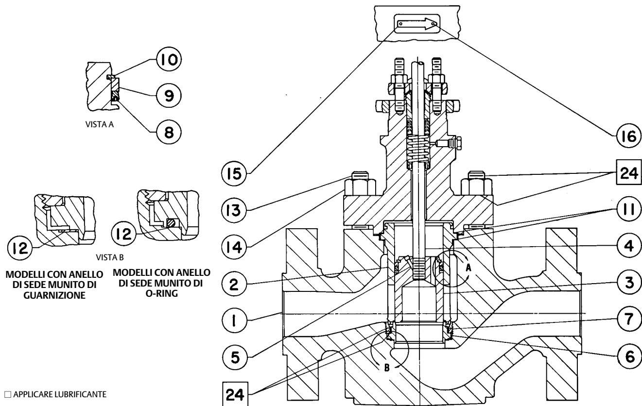
Figura 20. Valvola EHT Fisher
