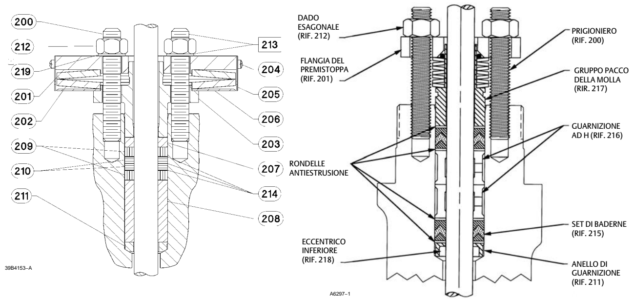
Sistema tipico di baderna HIGH-SEAL ULF
