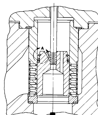
ECOULEMENT ELEMENTS INTERNES DE VANNE HPT, NPS 3-6, CAVITROL III 2 ETAGES
