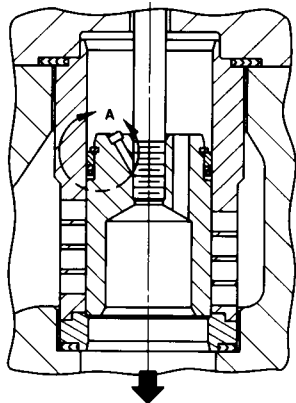
ECOULEMENT ELEMENTS INTERNES DE VANNES HPT ET HPAT (TOUTES TAILLES)
