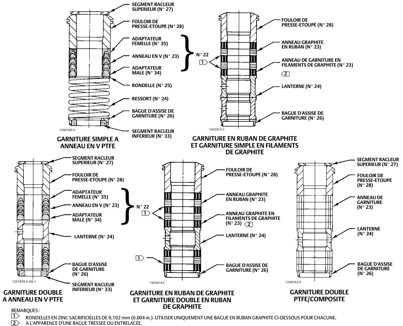
Figure 3. Configuration des garnitures d'étanchéité
