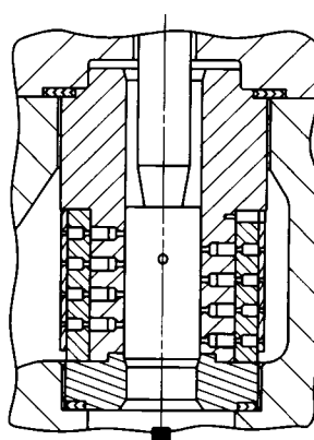
ECOULEMENT ELEMENTS INTERNES DE VANNE HPS, NPS 2, CAVITROL III 3 ETAGES
