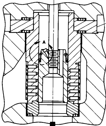
ECOULEMENT ELEMENTS INTERNES DE VANNE HPT, NPS 2, CAVITROL III 2 ETAGES
