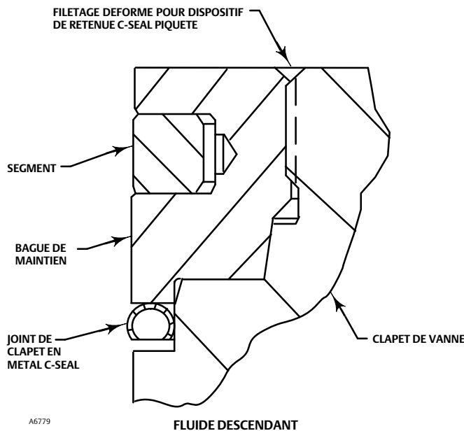
Figure 14. Piquetage du filetage du dispositif de retenue C-seal
