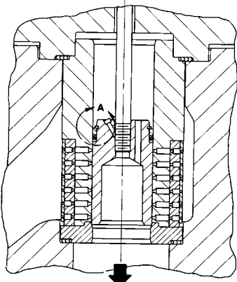
ECOULEMENT ELEMENTS INTERNES DE VANNE HPT, NPS 3-6, CAVITROL III 3 ETAGES
