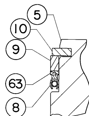
VANNES HPT, HPAT AVEC BAGUES ANTI-EXTRUSION PEEK
