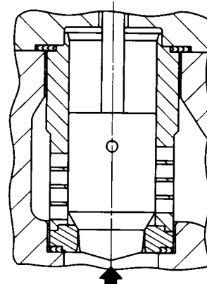
ECOULEMENT CLAPET MICRO-FORM VANNE HPS (NPS 2 UNIQUEMENT)
