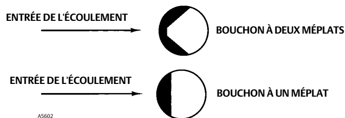
Figure 10. Orientation du clapet de vanne Micro-Flat
