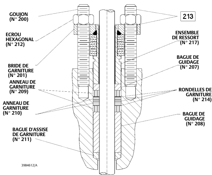
Garniture ENVIRO-SEAL avec garniture graphite ULF
