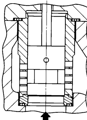
ECOULEMENT ELEMENTS INTERNES DE VANNE HPS, NPS 2-3
