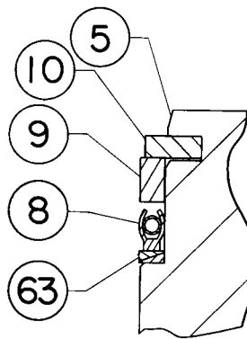
VANNES HPT, HPAT AVEC BAGUES ANTI-EXTRUSION PEEK
