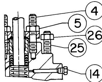
DETAIL DE LA VISSERIE DE L'ACTIONNEUR DU BOSSAGE D'ARCADE (EN OPTION POUR LES SERIES EH DE CORPS DE VANNE NPS 3, 4 ET 6) DE 127 MM (5 IN.)
