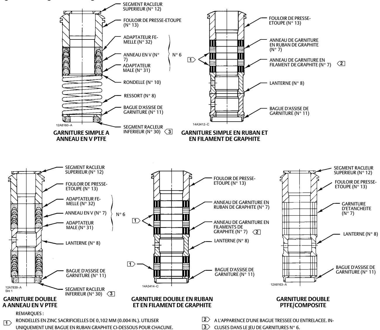
Figure 4. Configuration des garnitures d'étanchéité
