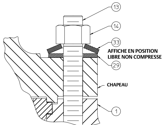
NPS 6 CL2500 NPS 8 ET PLUS TOUTES CLASSES ASME
