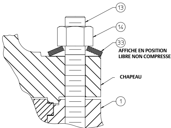
DE NPS 1-1/2 A NPS 4 TOUTES CLASSES ASME NPS 6 TOUTES CLASSES ASME SAUF CL2500
