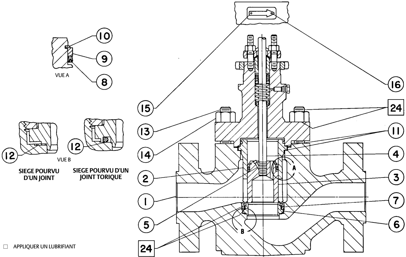
Figure 20. Vanne EHT de Fisher
