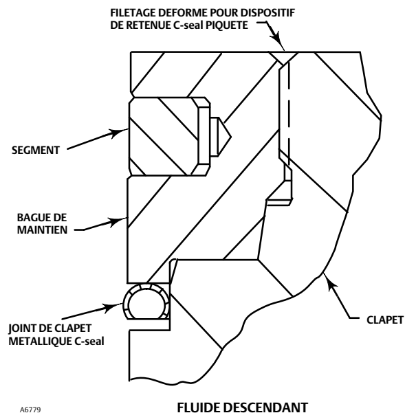
Figure 13. Piquetage des filetages de bague de maintien C-seal
