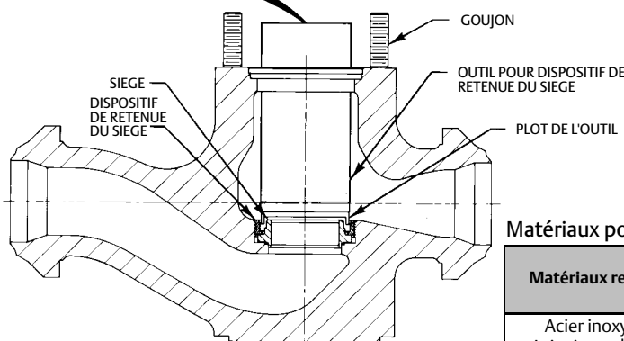
INSTALLATION DE L'OUTIL
