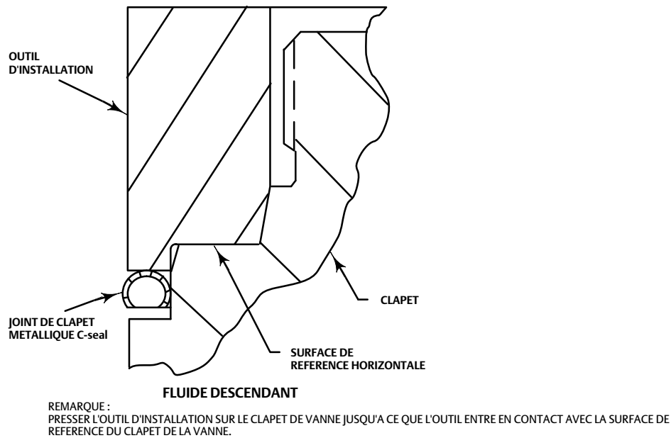
Figure 12. Installation du joint de clapet C-seal avec l'outil d'installation
