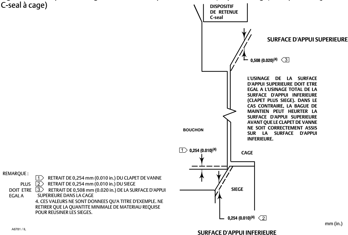
Figure 15. Exemples d'usure des surfaces de portée inférieure (clapet au siège) et supérieure (joint C-seal à cage)
