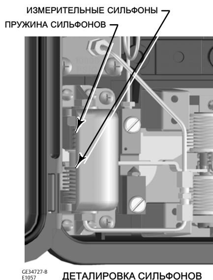
Рис. 5. Детализовка сильфонов
