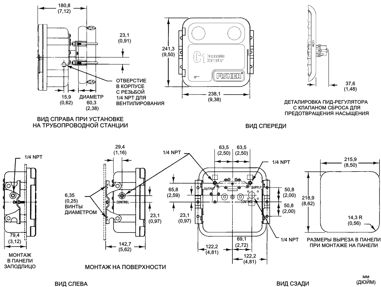
Рис. 8. Размеры
