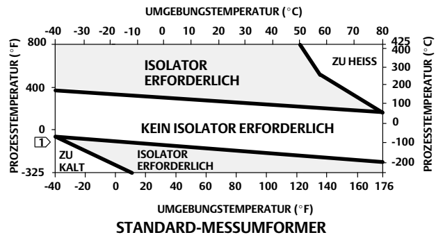
Abbildung 1. Richtlinien für den Einsatz des optionalen Temperaturisolators
