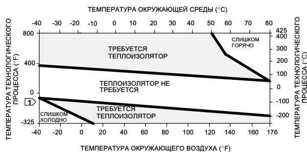
Рисунок 1. Основные принципы применения дополнительного узла теплоизолятора
