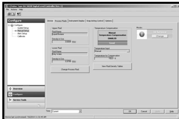
Figure 2. AMS Suite : Écran de configuration d'Intelligent Device Manager
