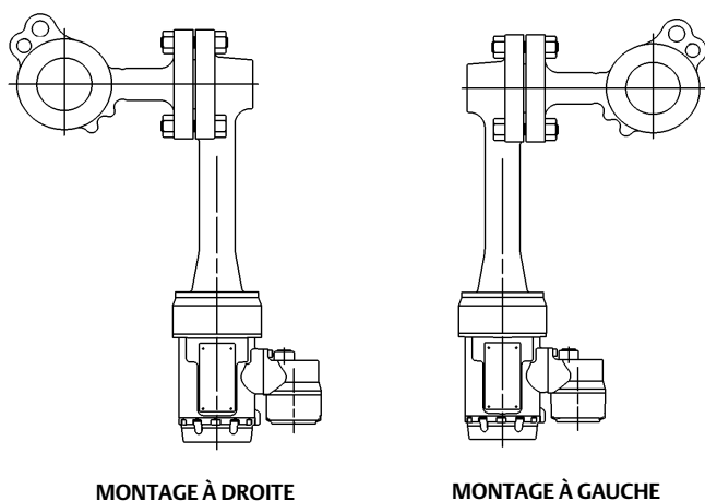
Figure 11. Positions de montage - Entre brides (cage fournie par le client)
