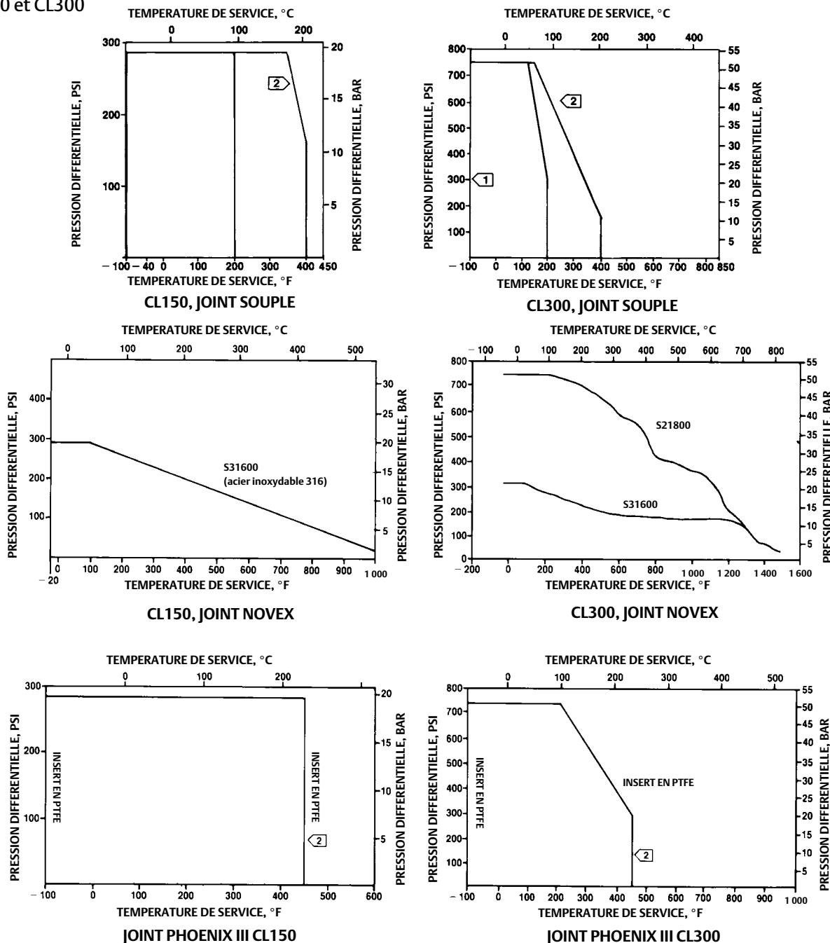
Figure 4. Limites de pression/température maximum pour le joint souple, le joint NOVEX et le joint Phoenix III, CL150 et CL300
