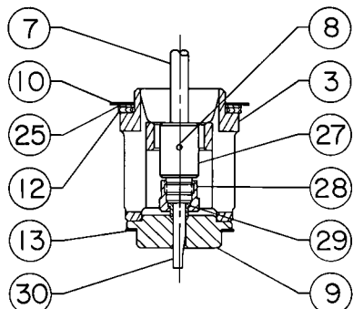
VOŽTUVO UŽDORIS „MICRO-FLUTE“, 6,4 mm (0,25 COL.) SKYLĖS SKERSMUO
