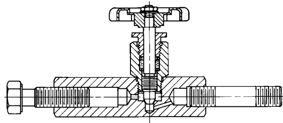
TEPTUVAS SU ATSKYRIMO VOŽTUVU
