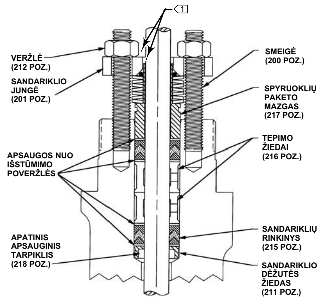
7 pav. Tipinė sandariklių „ENVIRO-SEAL“ sistema su PTFE sandarikliu
