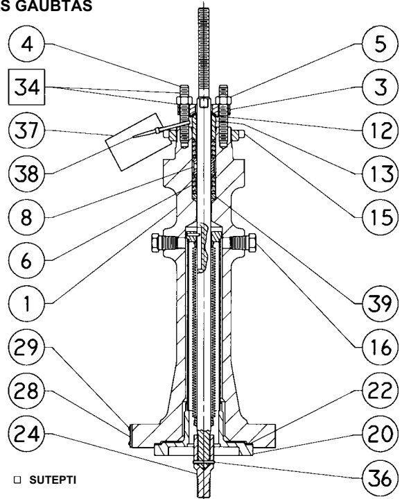
GAUBTAS SU SILFONINIŲ SANDARIKLIŲ „ENVIRO-SEAL“
