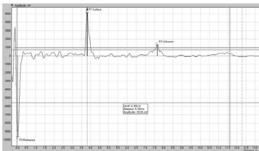
График 1. График эхо-сигнала
