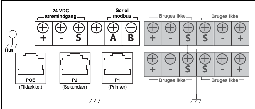
Figur 1. 1420 Klemmeblokdigram
