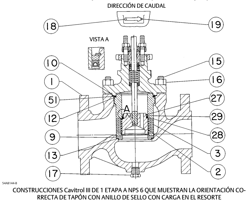
Figura 20. Detalles de válvulas ET Fisher NPS 8 y Cavitolr III con tapón de drenaje opcional
