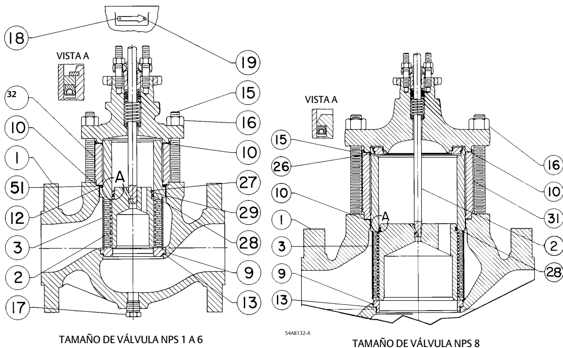
TAPÓN Y ANILLO DE SELLO CON CARGA EN EL RESORTE QUE MUESTRAN LA ORIENTACIÓN CORRECTA PARA LA JAULA Cavitolr III DE DOS ETAPAS
