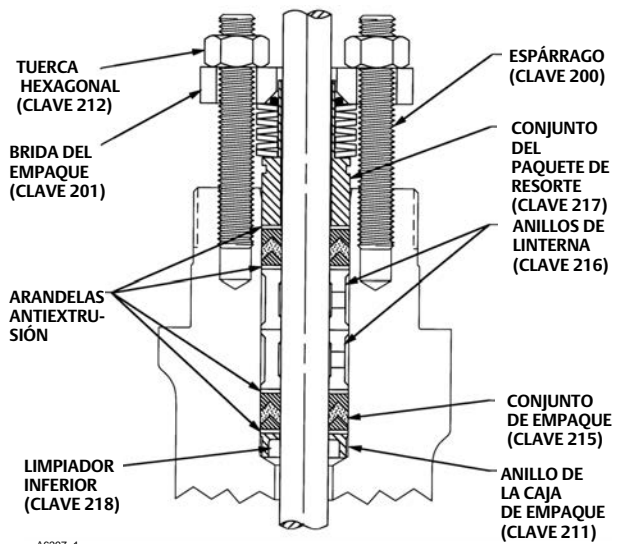
Figura 11. Sistema de empaque ENVIRO-SEAL típico con empaque de teflón
