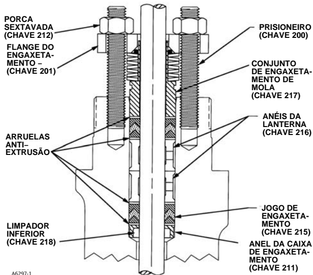
Figura 11. Sistema típico de engaxetamento ENVIRO-SEAL com engaxetamento de PTFE
