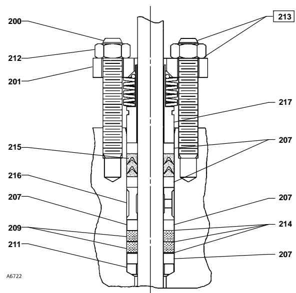
Figura 13. Sistema típico de engaxetamento ENVIRO-SEAL com engaxetamento duplo
