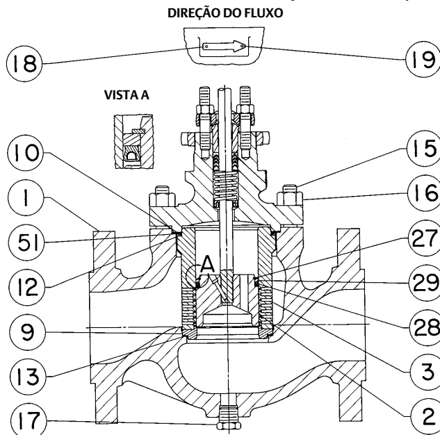
CONSTRUÇÕES DE UM ESTÁGIO Cavitrol III A NPS 6 MOSTRANDO A ORIENTAÇÃO CORRETA DO BUJÃO COM ANEL DE VEDAÇÃO ACIONADO POR MOLA
