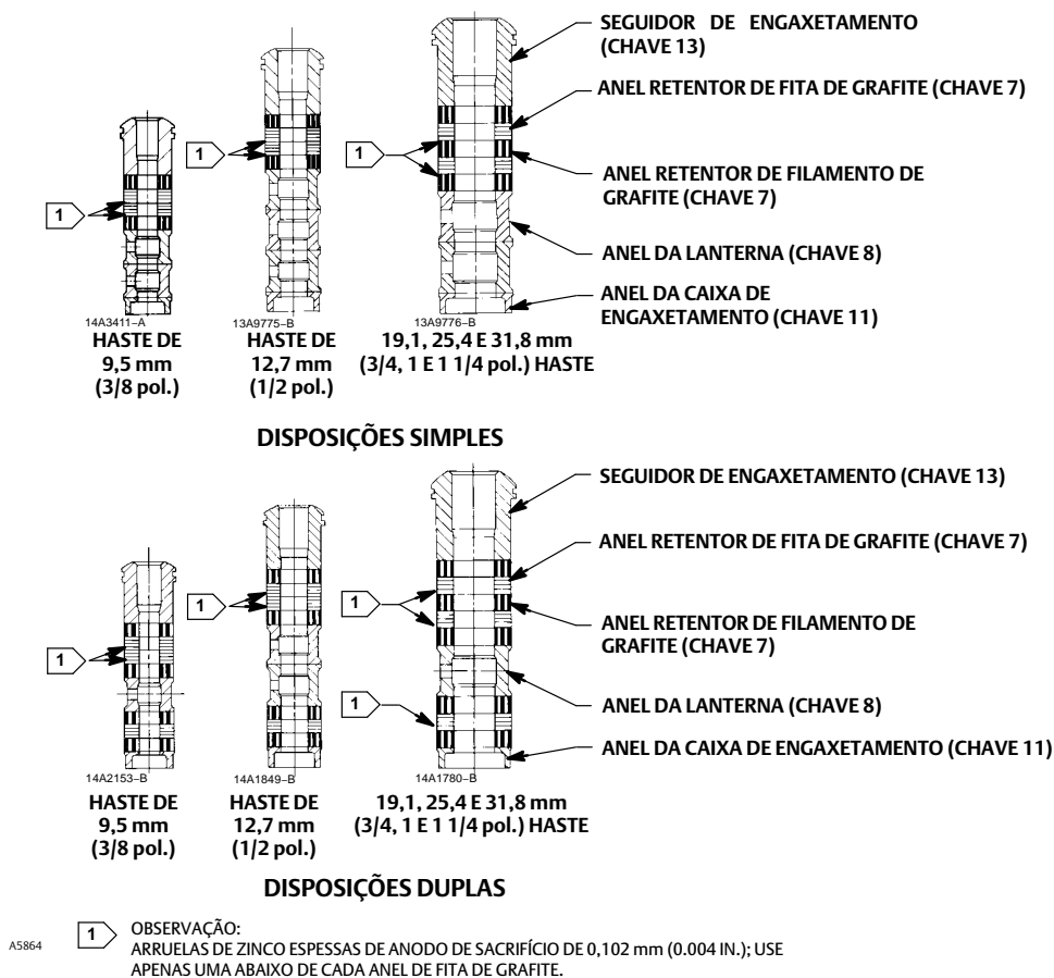
Figura 5. Detalhe do engaxetamento de fita de grafite/filamento para capôs simples e de extensão
