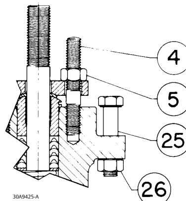
DETALHE DE 127 mm (5 pol.) FIXAÇÃO DO ATUADOR DA PROTUBERÂNCIA DO GARFO
