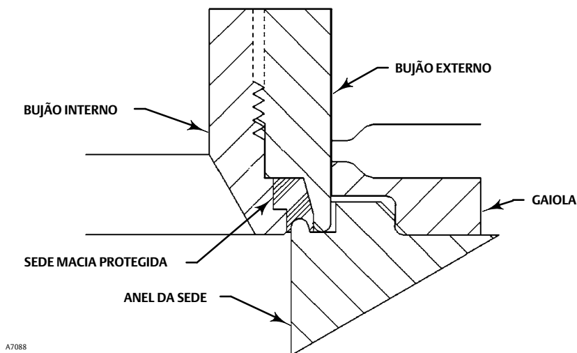
Figura 6. TSO (sigla em inglês que significa: guarnição de fechamento hermético), detalhe da sede macia protegida
